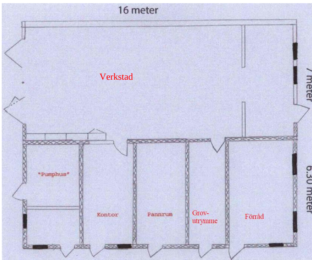
Bild 23. Schematisk skiss över garage/ verkstadslokal med inritad inre vägg.
