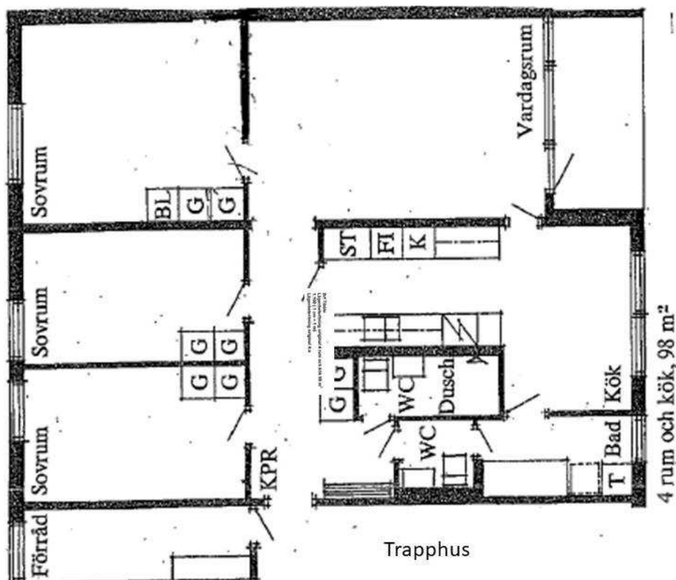
Figur 5. Originalritning skickad av fastighetsförvaltaren Mikael Weidenhag.
