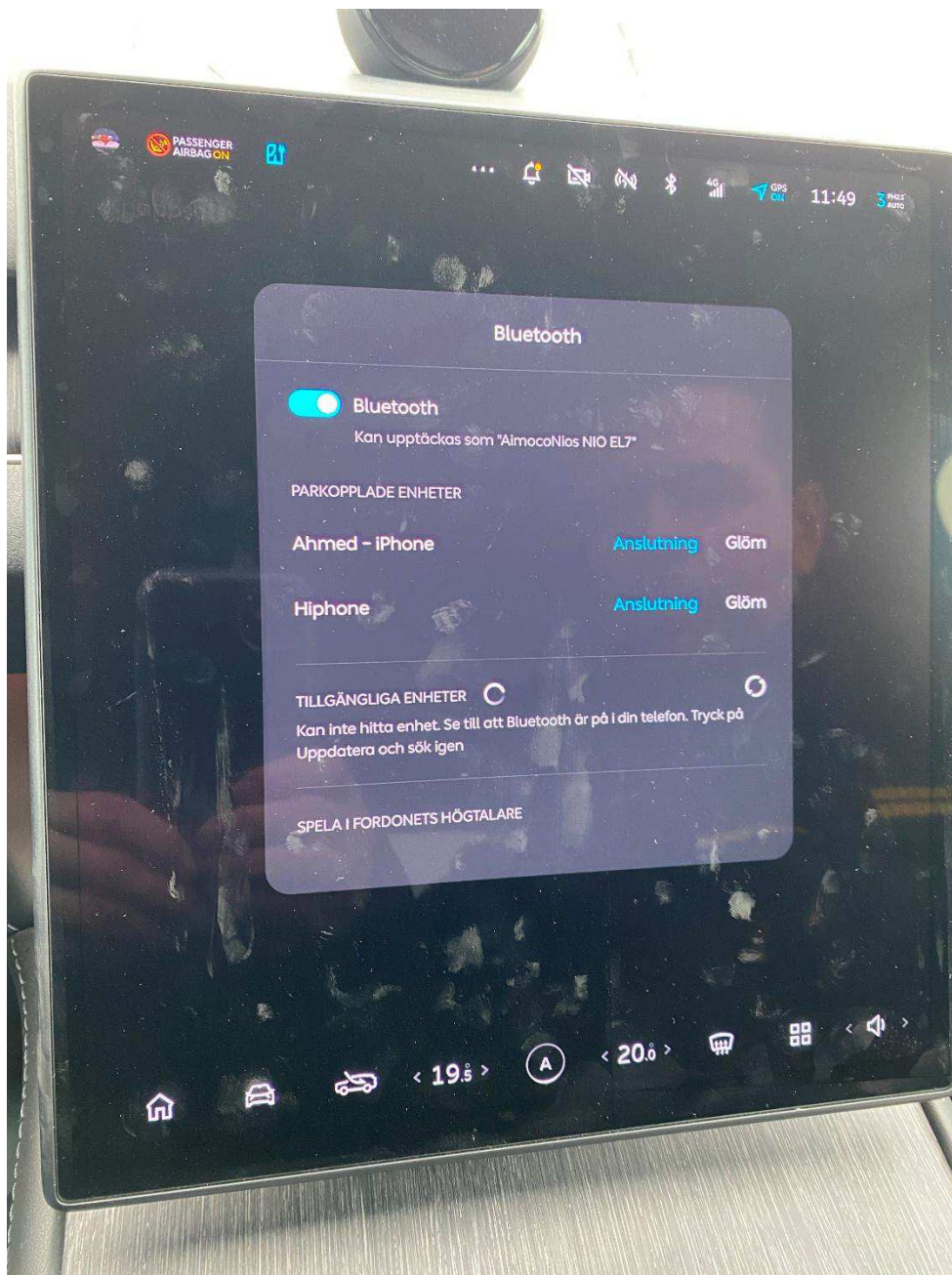
Bluetooth uppkopplingar
