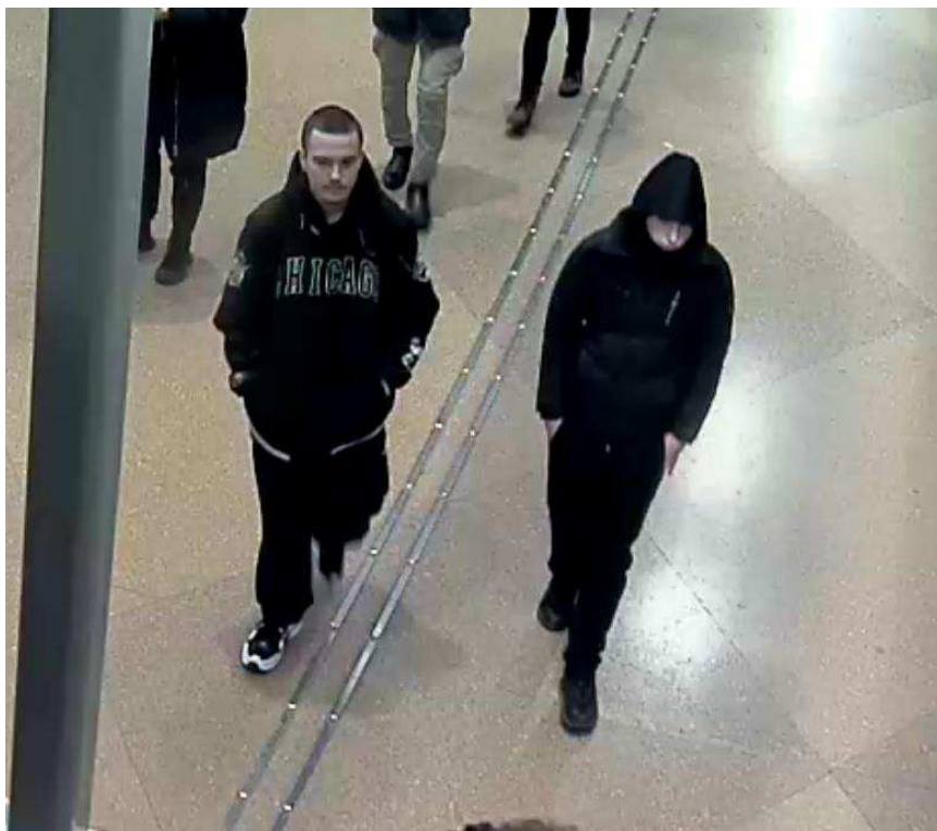
Sci-P106, 21:20:47
