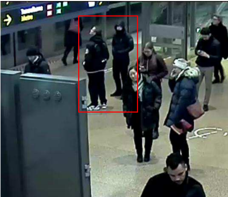
Sci-P107, 21:15:00
