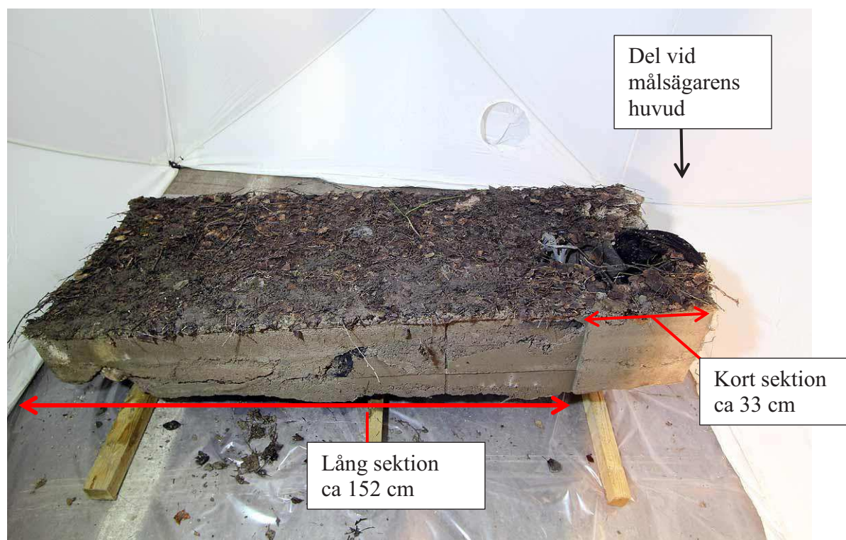
Figur 1. Betongblocket. Måttangivelser.
