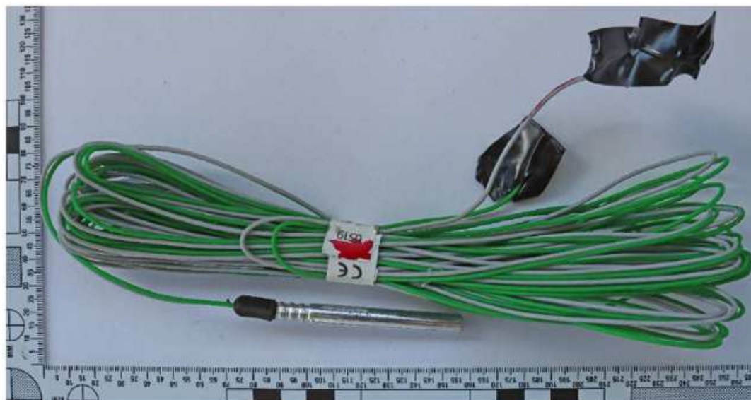
Bild 1: Beslagtagen elsprängkapsel.
