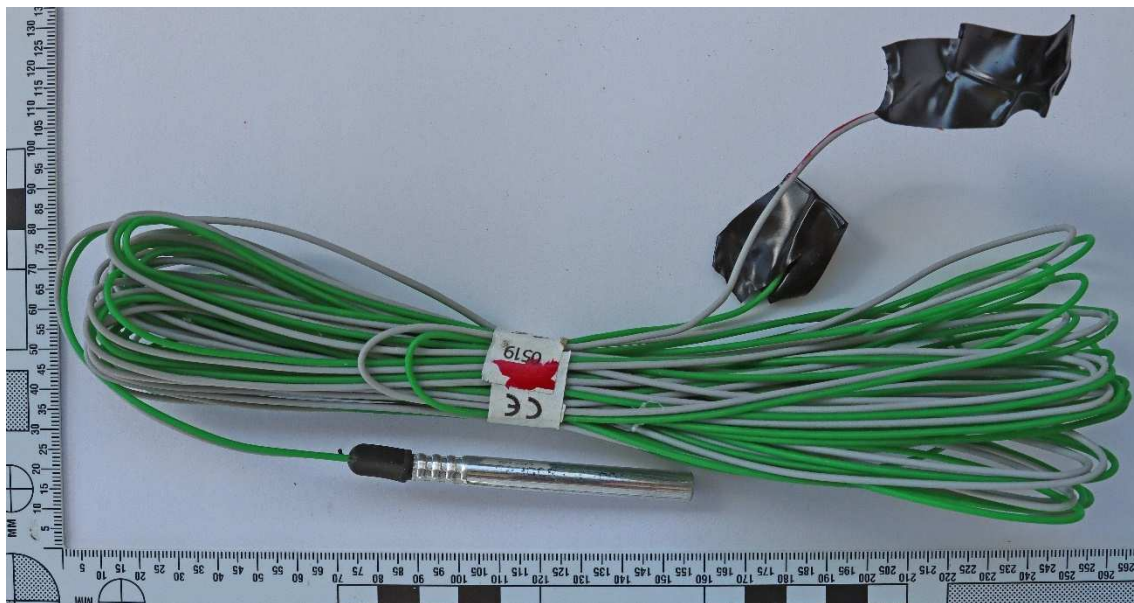
Bild 1: Beslagtagnen elsprängkapsel.
