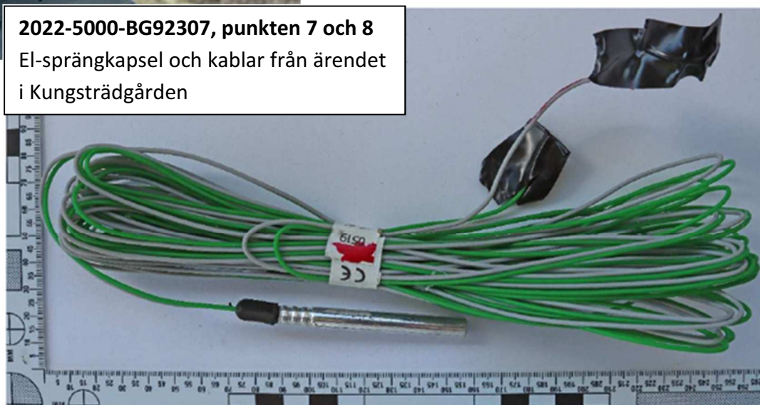
Bild 1: Beslagtagn elsprängkapsel.
