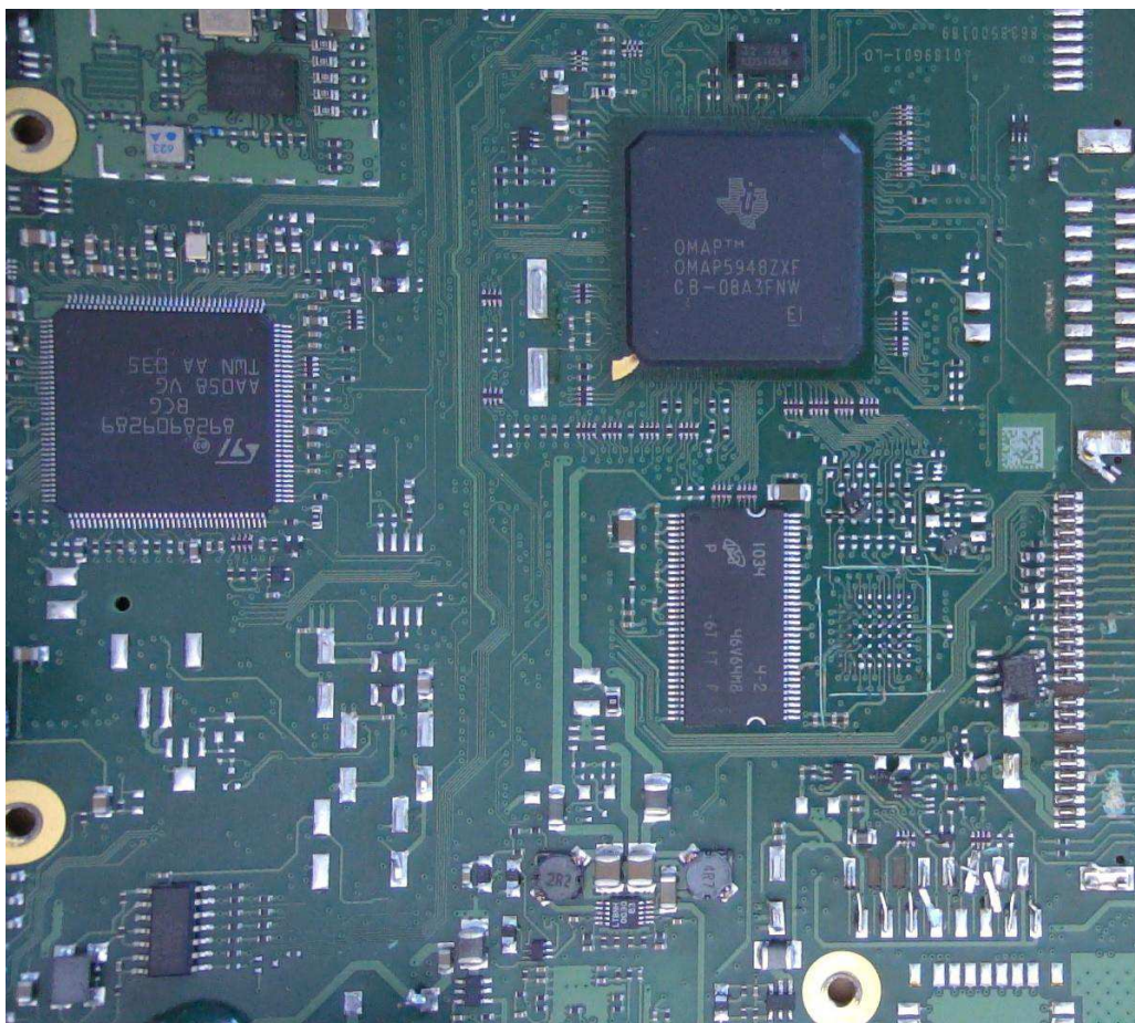
Bild på kretskort från bilen infotainmentenhet
