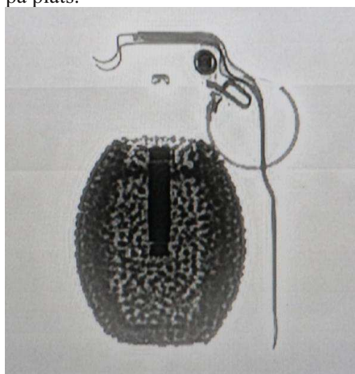
Figur 11. Röntgenbild av handgranaten (G010-G012) i intakt skick.
