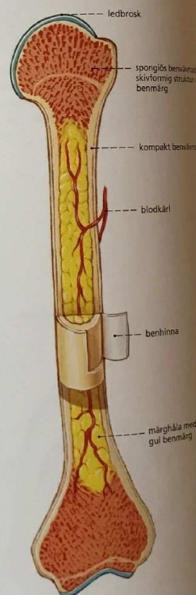
Fig. 21 Uppbyggnad av ett ben (överarmsbenet). I partierna nära en led (nära överst och underst) är benvävnaden ordnad i skivor och har ett poröst spongiöst utseende (av latin spongiosa som betyder [svampig/svampig]). Skivorna ger hög motståndskraft mot tryck och spänning.
