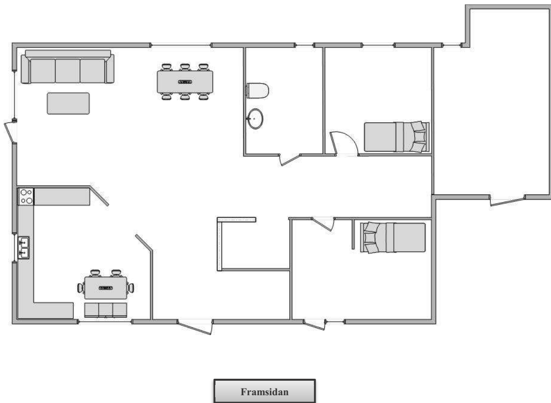
Figur 17. Schematisk planritning på markplanet av huset.
