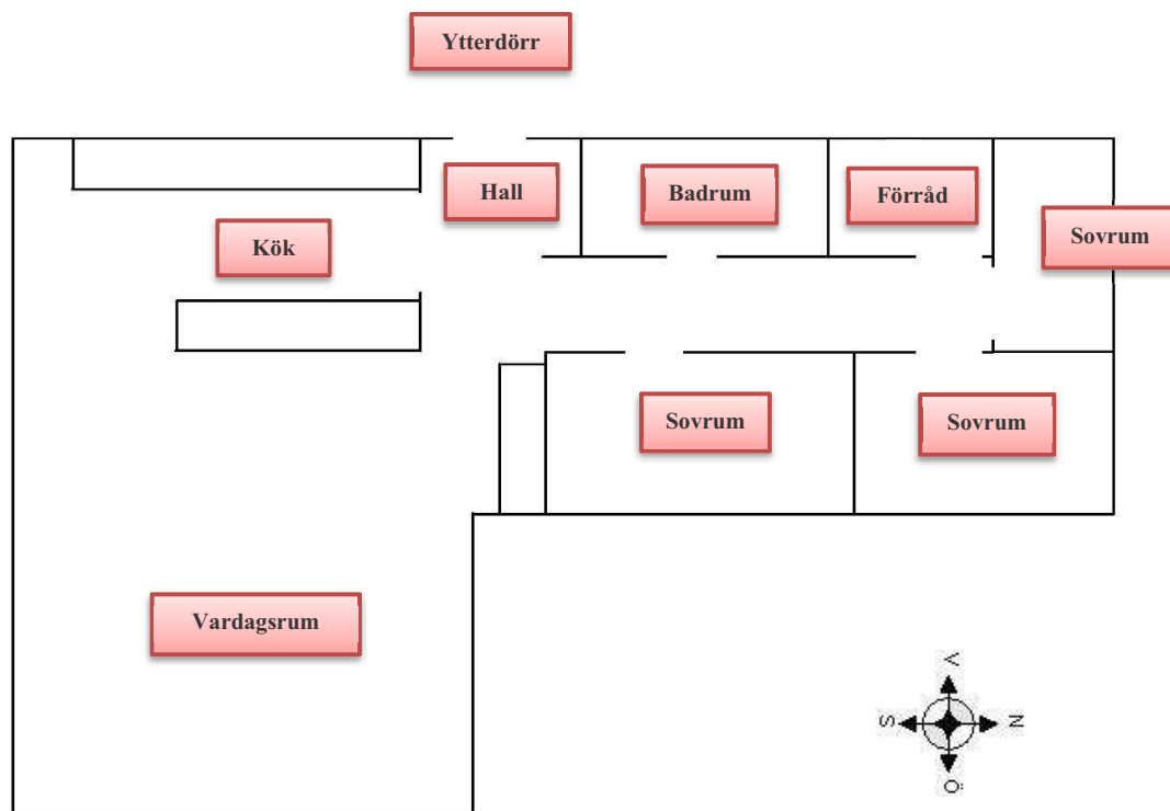
Figur 10. Schematisk planritning.
