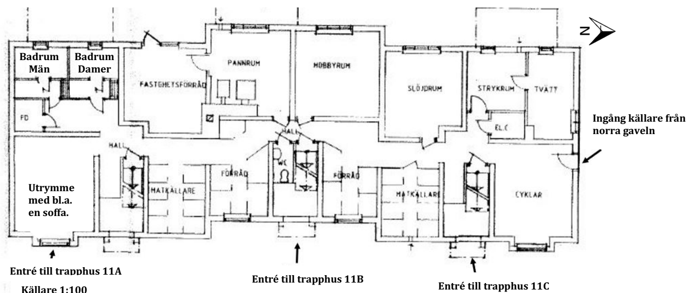
Figur 5. Planritning över källaren Fäbodvägen 11, Horndal. Planritningen inlämnad av fastighetsägaren Peter Höglund 2023-08-05. Redigering av vissa rum har gjorts av kriminaltekniker Inga-Lill Persson 2023-08-08.
