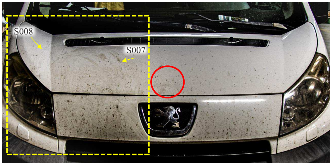
Figur 3. På huvens vänstra sida iaktogs det som bedömdes vara drag/släp/styrspår (S007-S008). Området är markerat med en streckad rektangel. Mitt på huven, ovanför Peugeotmärket, iaktogs en inbuktning i plåten. Inbuktningen är markerad med en cirkel.
