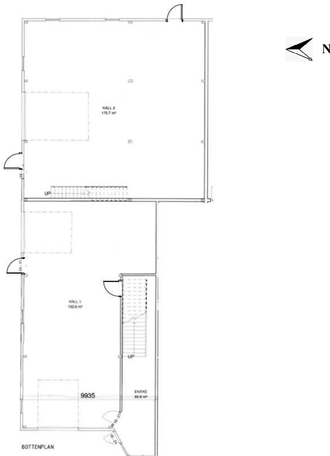
Figur 5. Norra delen av huset, bottenplanet. Ritning erhållen av Hedemora kommun 2023-10-24. Ritningen kompletterad av Olov Bokefors då den inte riktigt överensstämde med faktiska förhållanden.
