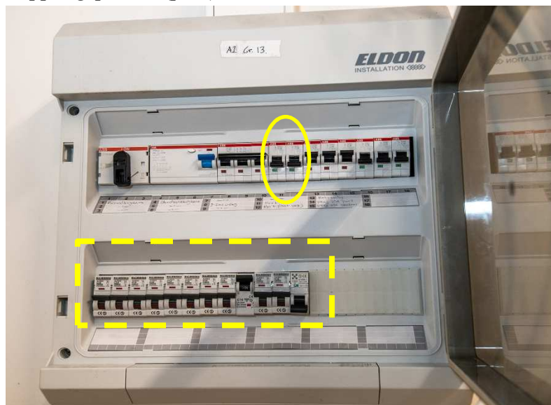
Figur 15. Elcentralen. Säkringarna till fordonshallens portar ses fränkopplade och inringade med gult i den övre kopplingsplinten. Enligt den elektriker som kopplade bort elen ur centralen så var dessa initialt fasttejpade i fränkopplat läge. Den gulstreckade ramen markerar kopplingsplinten till vilken all el till odlingsrummet var kopplad.
