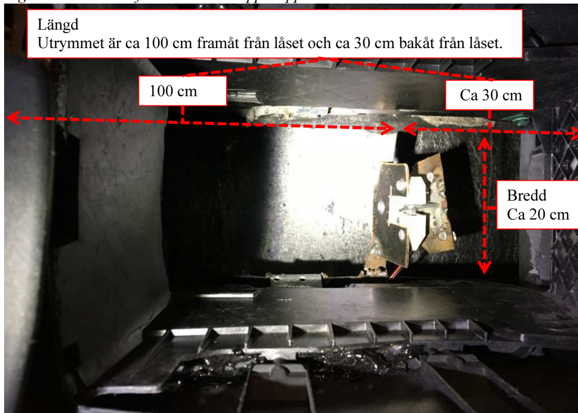
Figur 5: Låsdetaljer satt kvar under det bortbrutna innerfacket.
