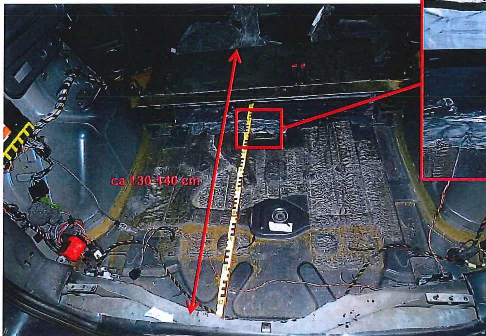
Bild 54. Lönnutrymmet i fordonet var ca 130-140 cm långt var av ca 50 cm av utrymmet finns under det bakre sätet. Se pil och förstoring.
