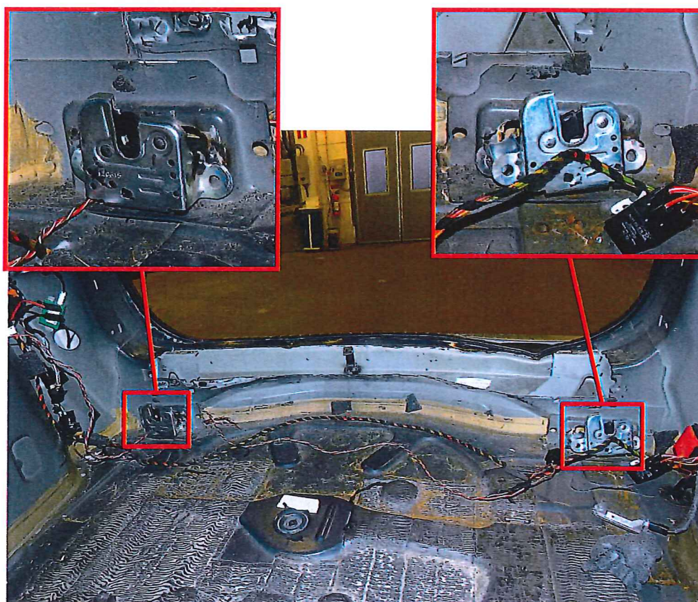
Bild 51. Luckan till lönnutrymmet låstes med två låsinsatser.
