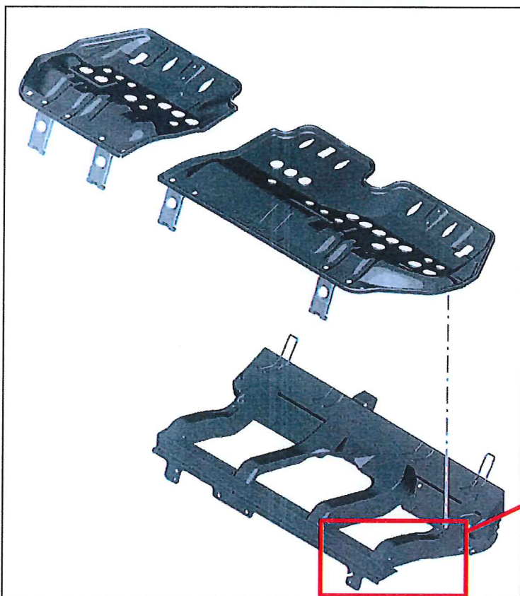
Bild 47. Sprängskiss över "Bakre sätessomme" för det undersökta fordonet.
