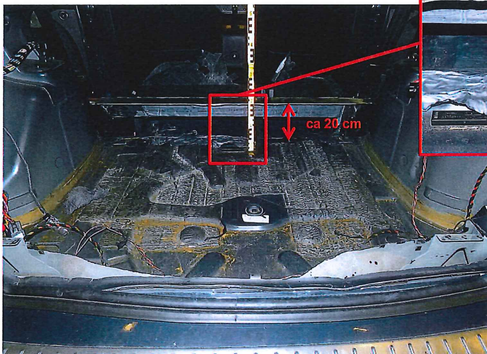
Bild 55. Lönnutrymmet i fordonet var ca 20 cm högt. Den del av utrymmet som går under baksätet är något lägre. Se pil och förstoring.
