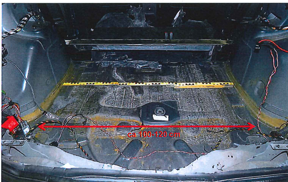
Bild 53. Lönnutrymmet i fordonet var ca 100-120 cm brett. Den del av utrymmet som går under baksätet är något mindre. Se pil.
