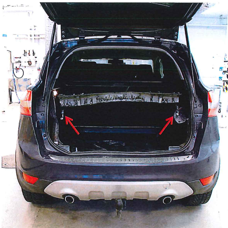
Bild 50. Luckan till lönn- utrymmet hade två fastsvetsade krokar. Se pil. Krokarna låstes fast de elektroniskt styrda låsen. Se bild 51-52.
