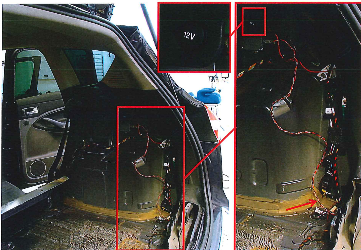
Bild 52. Låsen var elektroniskt styrda och kopplade till ett 12V-uttag i bagageutrymmet. Slöts strömmen i detta uttag kunde låsen öppnas. Se pil och förstoringar.
