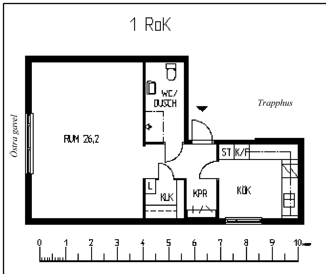
Bild 3. Lägenhet ritning. Ritningen skickad av Heimstaden, ägare av byggnaden.
