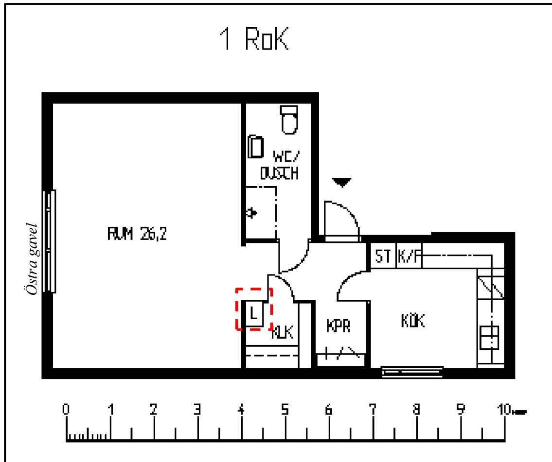
Bild 3. Lägenhet ritning. Ritningen skickad av Heimstaden, ägare av byggnaden. Den aktuella garderoben är markerad i ritningen.
