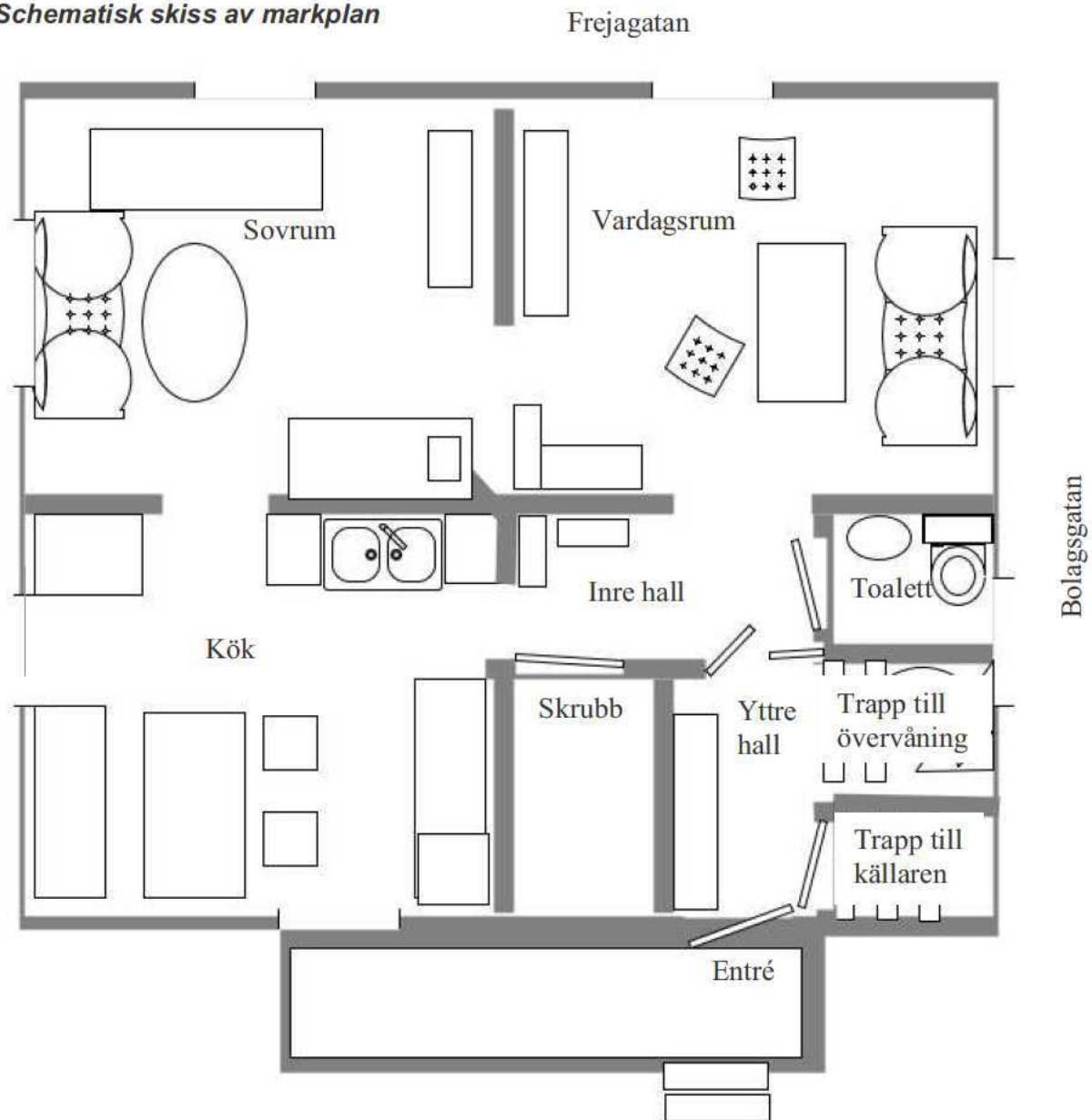
Bild 12. Schematisk skiss av villans markplan upprättad av Carola Mickelsson.
