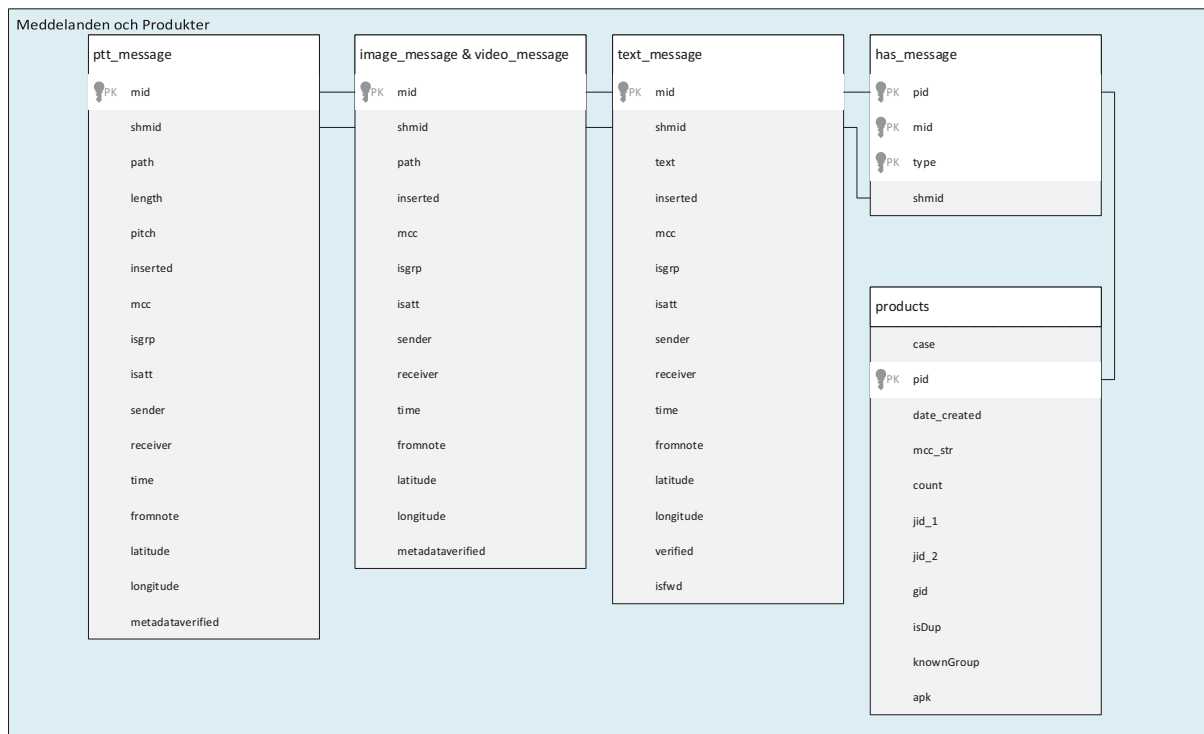
Figur 1 Databasstruktur meddelanden
