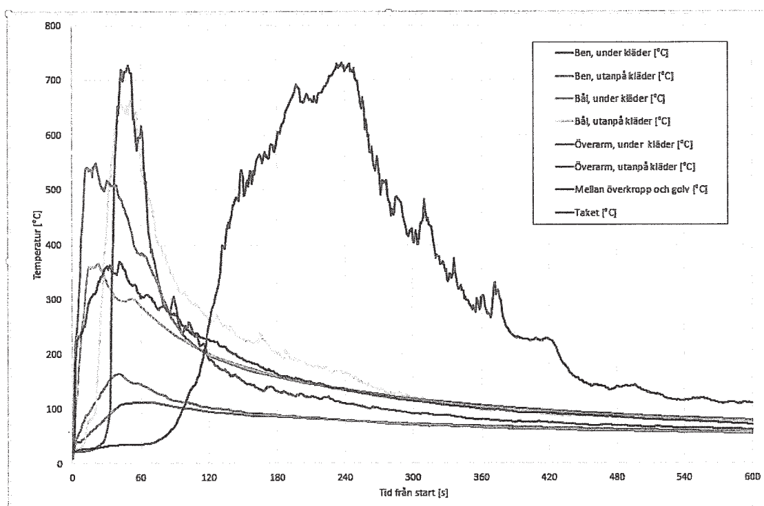
Brandförsök 2.
