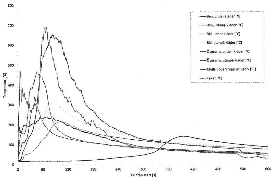
Brandförsök 1.
