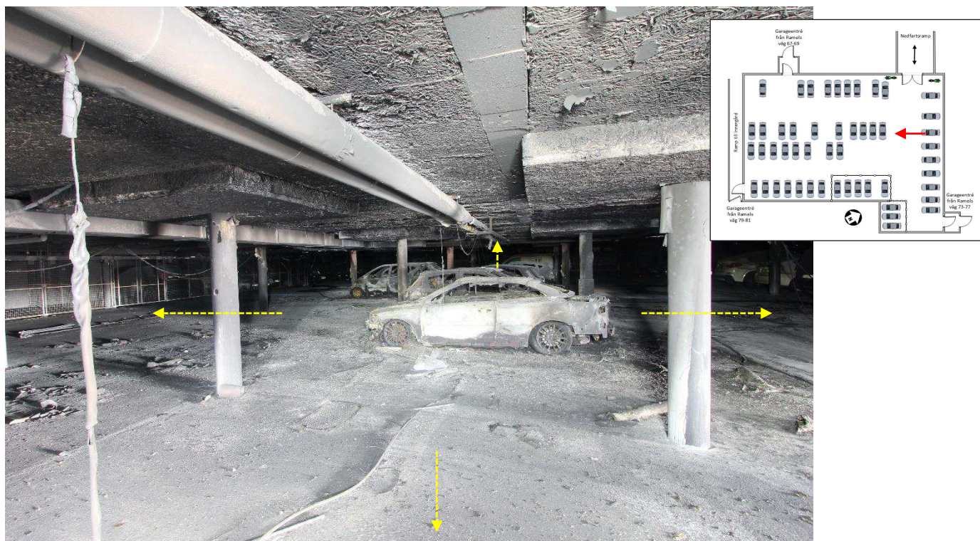
Figur 10. Garagets mitt del. Avtagande brandskador mot garagets ytterväggar visualiseras med streckade gula pilar.
