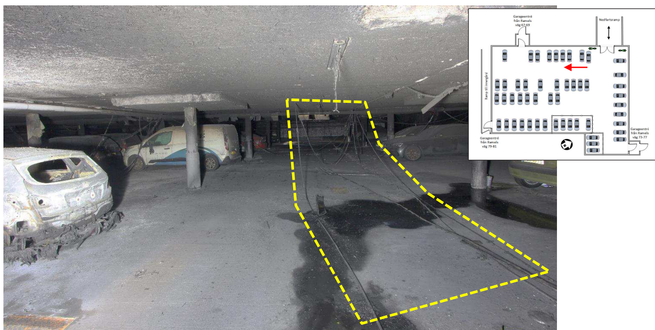
Figur 11. Översikt bild över södra delen av garaget. Brandskadade kablar inom markeringen.
