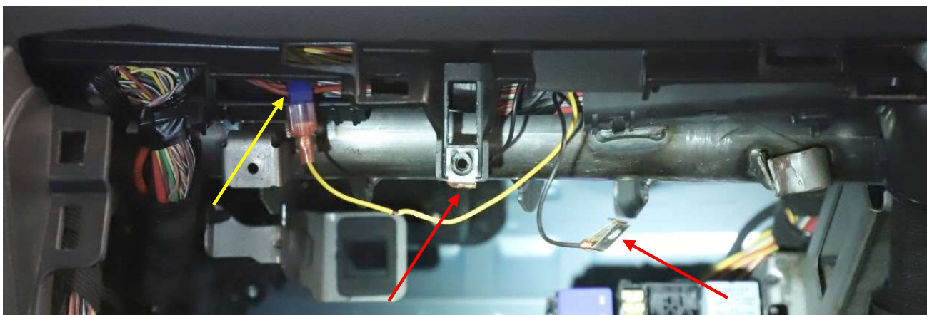
Bild 21. Bakom handskfacket återfinns den gula och de svarta sladdar som löper från gömmornas lås. Den gula är påkopplad på fordonets befintliga elsystem (gul pil) medan den ena svarta är fastklämd runt skruvens fäste och den andra hänger löst bredvid (röda pilar).
