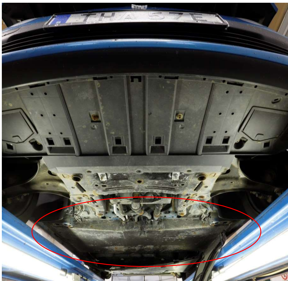
Bild 24. När de främre kåporna monterats bort blir det påsvetsade lönnutrymmet synligt. Denna del tillhör inte bilens originalutförande.
