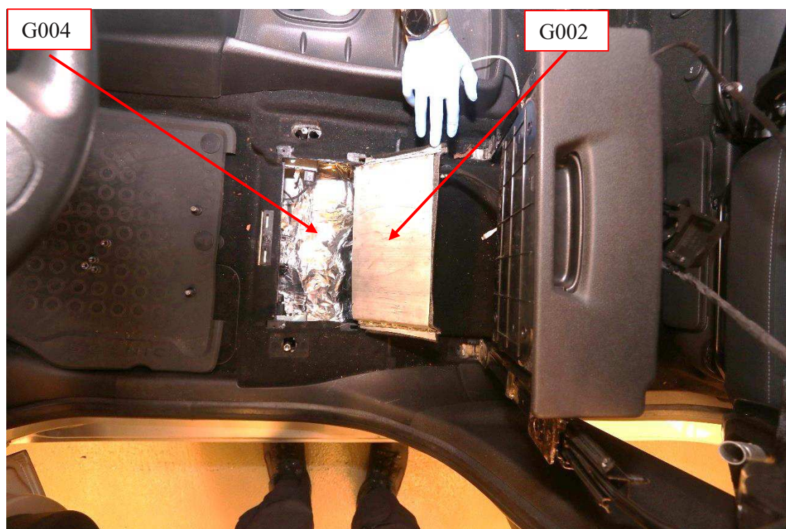
Figur 12: Visar luckan G002) i golvet under förarsätet, öppet läge när förarstolen är bortmonterad. Fordonsisoleringsmatta (G004) markerad.
