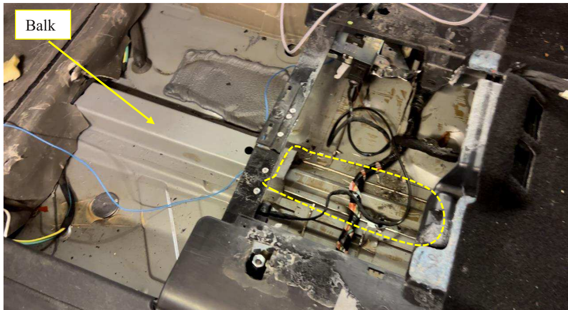
Figur 14: Visar att balk under sätet har kapats av och tagits bort för att skapa utrymme, markerat som streckat område.
