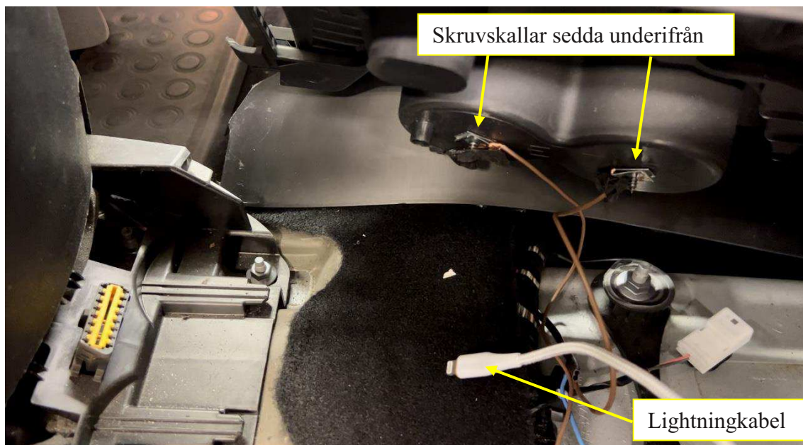
Figur 20: Visar skruvskallar i mittkonsolens drickahållare, sedda underifrån.
