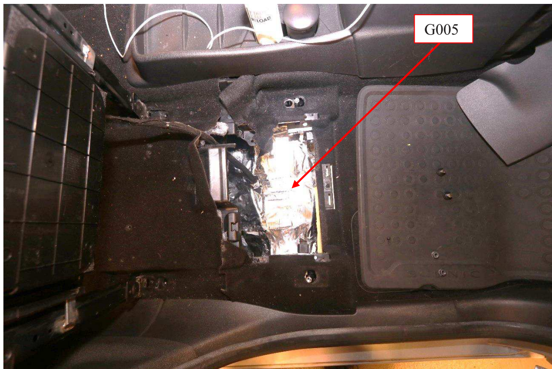
Figur 18: Visar hålet i golvet under passagerarsätet fram (luckan demonterad), öppet läge när passagerarstolen är bortmonterad. Fordonsisoleringsmatta (G005) markerad.
