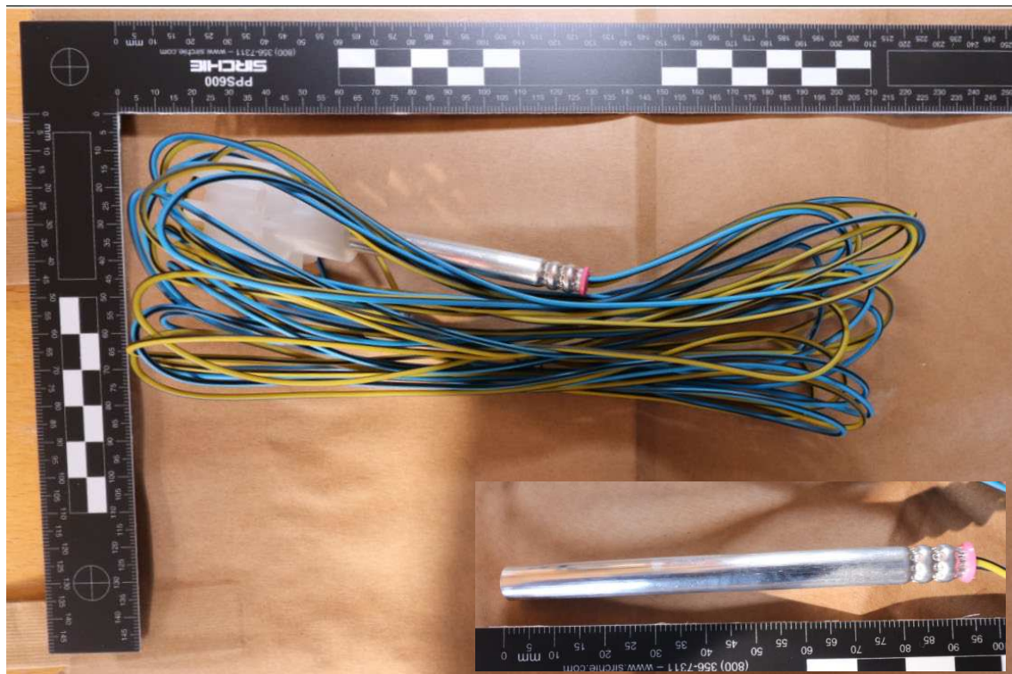
Figur 2. Elsprängkapsel utan emballage.
