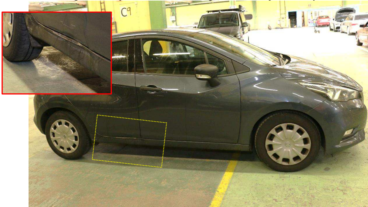
Figur 6. Bilens högra sida. Markering visar var skadan på balken under bakdörren observerades. Infälld bild visar skadan.
