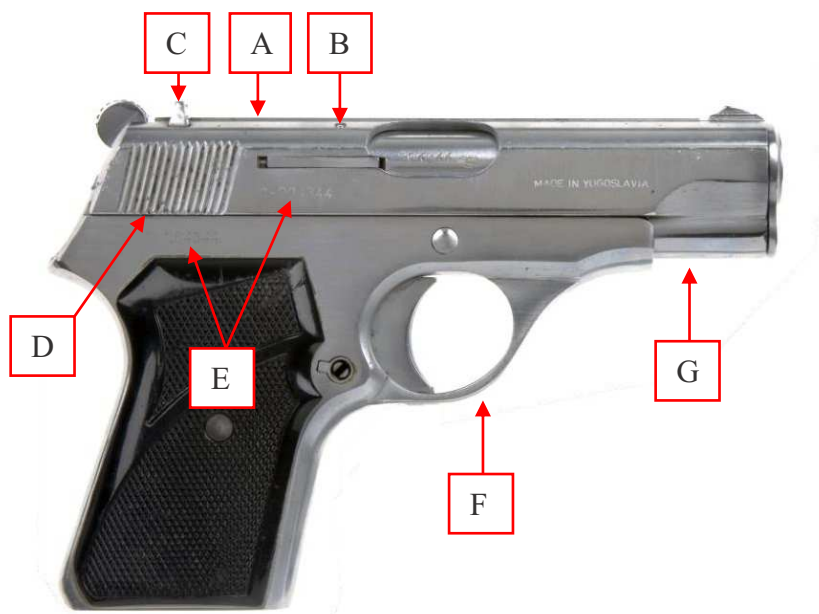
Bild 4. Skarp pistol av märke och modell Crvena Zatava/Zastava Arms M70 i kaliber 7,65 mm Browning (.32 Auto, .32 ACP). På bilden har pistolens spång (A), låssprinten till utdragaren (B), siktet (C), mantelgreppet (D), placeringen av tillverkningsnumren på stommen och manteln (E), formen på varbygeln (F) samt formen på mantelns främre del (G) markerats.
