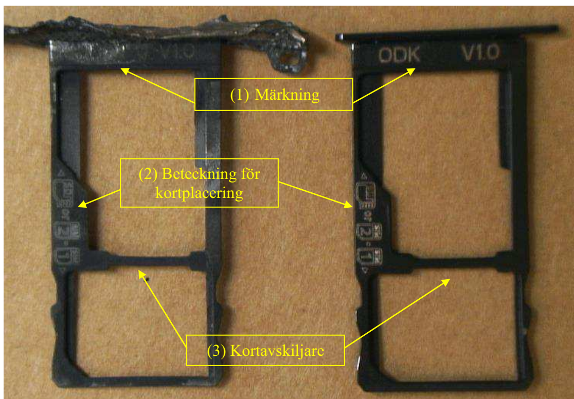
Bild 2 Simkorthållare 2020-5000-BG44267-5 (vänster) och BQ Aquaris X2 (höger)
