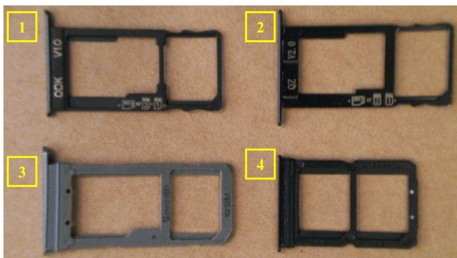
Bild 1 Simkorthållare för (1) BQ Aquaris X2, (2) BQ Aquaris X, (3) Samsung S7 Edge, (4) Huawei Mate 20 Pro
