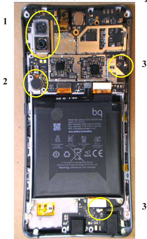
Bild 3 BQ Aquaris X2
