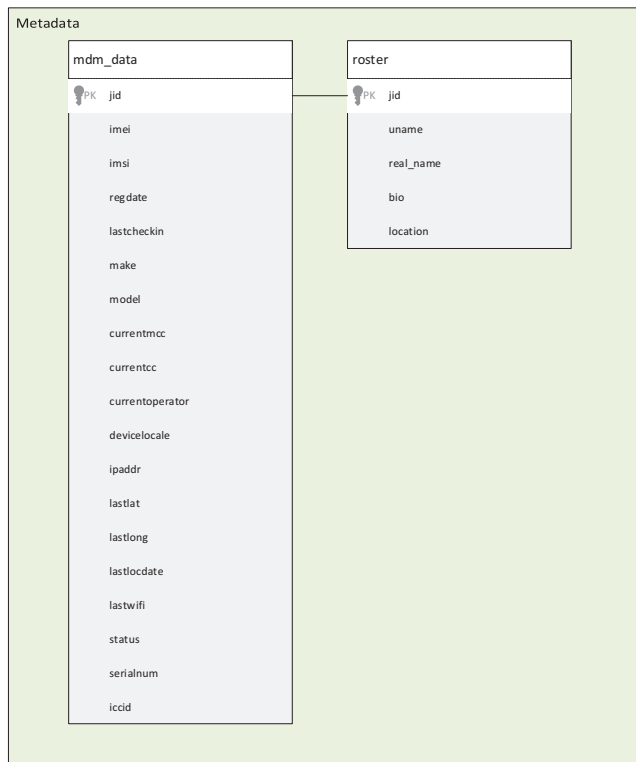
Figur 2 Databasstruktur metadata
