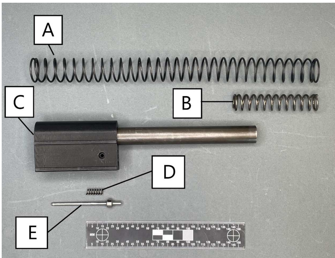
Figur 1. A, rekylfjäder, B buffertfjäder, C slutstycke, D tändstiftsfjäder, E tändstift. Dessa delar gör vapnet 2022-5000-BG141517-10 komplett.
