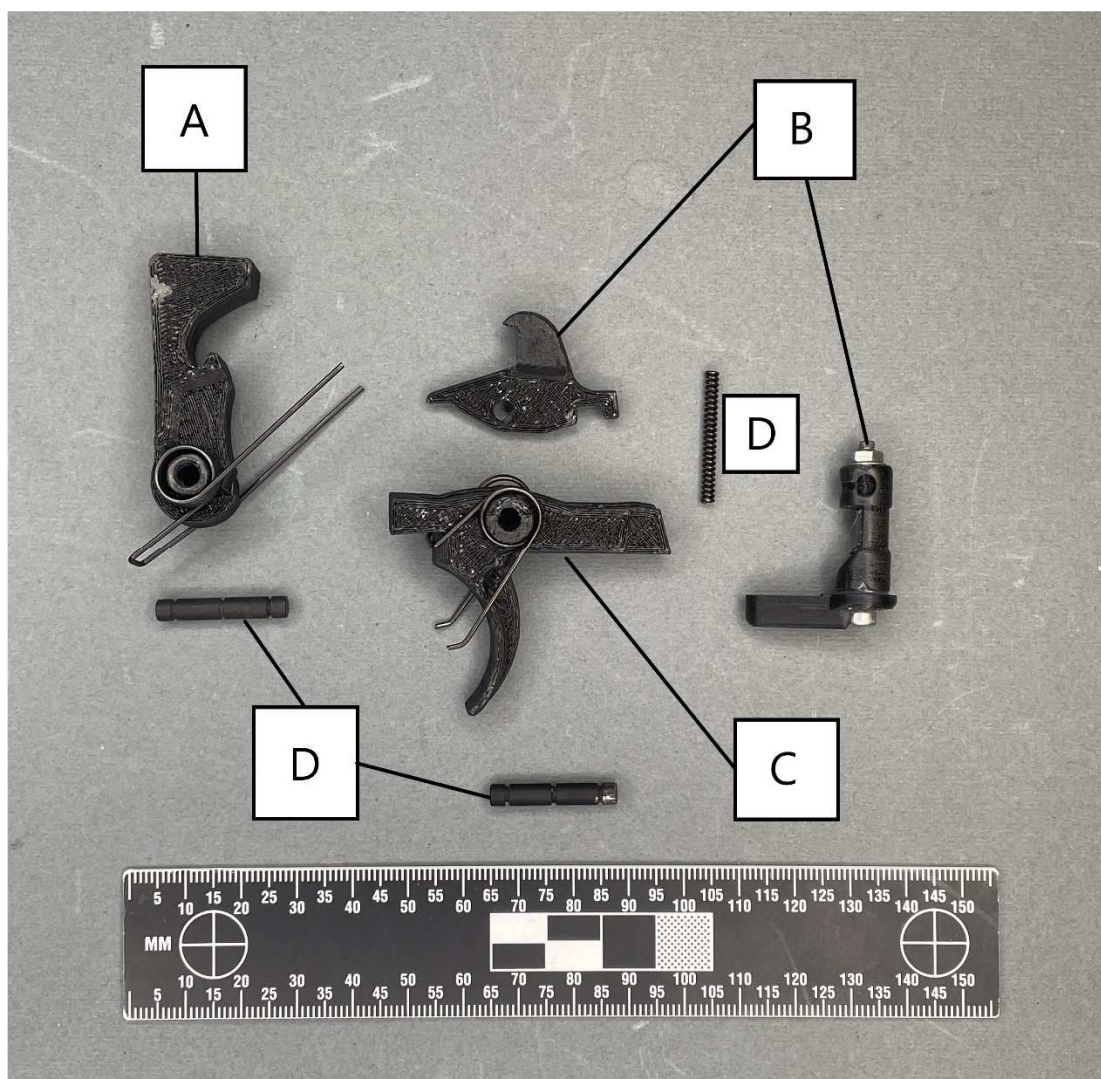
Figur 7. A- hane, B- avtryckarstäng och omställare, C- avtryckare, D- sprintar och fjäder.
