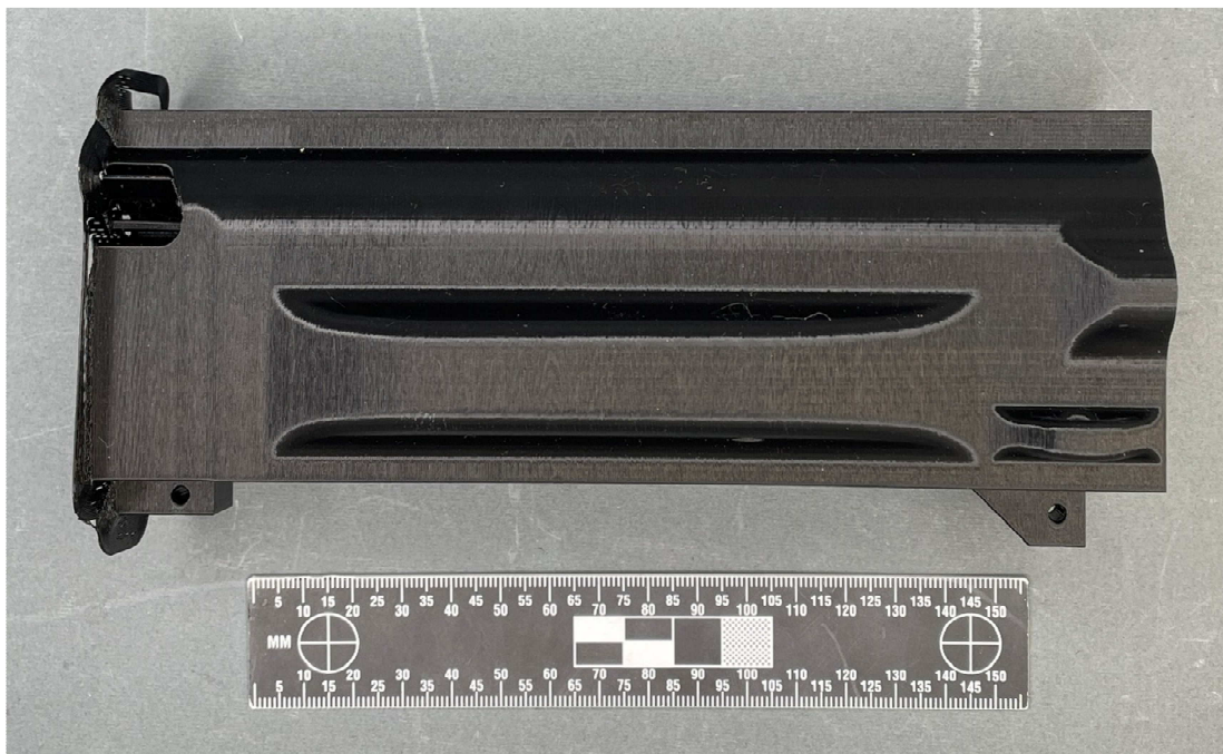
Figur 2. Låda till FGC-9 MKII, 2022-5000-BG141517-81
