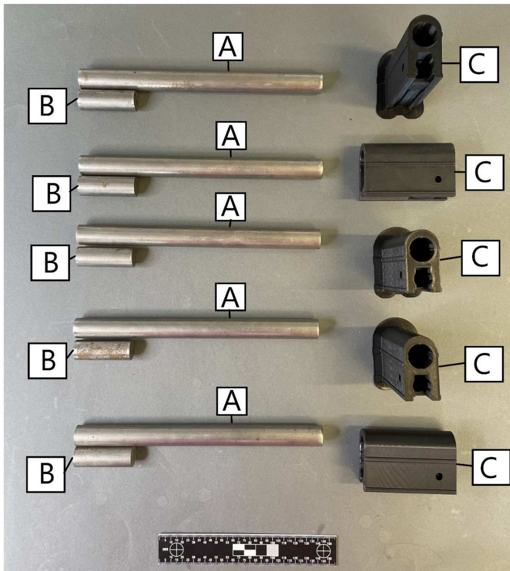
Figur 10. Material för slutstycken.
