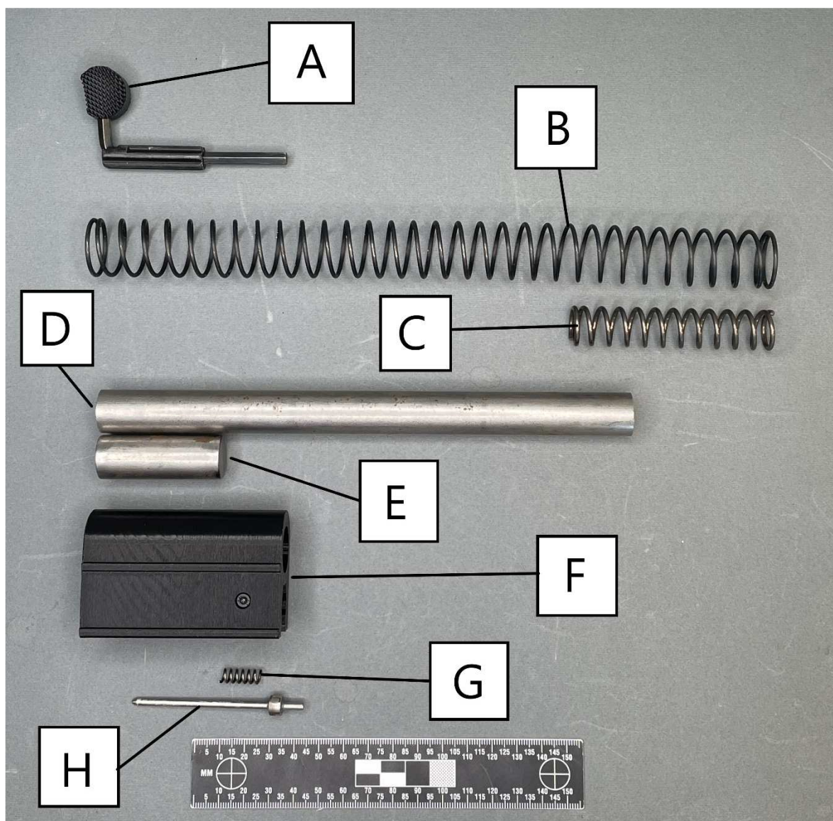
Figur 4. A- manöverhandtag, B- rekylfjäder, C- buffertfjäder, D- slutstycksstång, E- stötbotten, F- slutstyckshus, G-tändstiftfjäder och H-tändstift.
