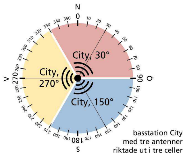
Bild 2. Illustration av basstations antenner och riktning.
