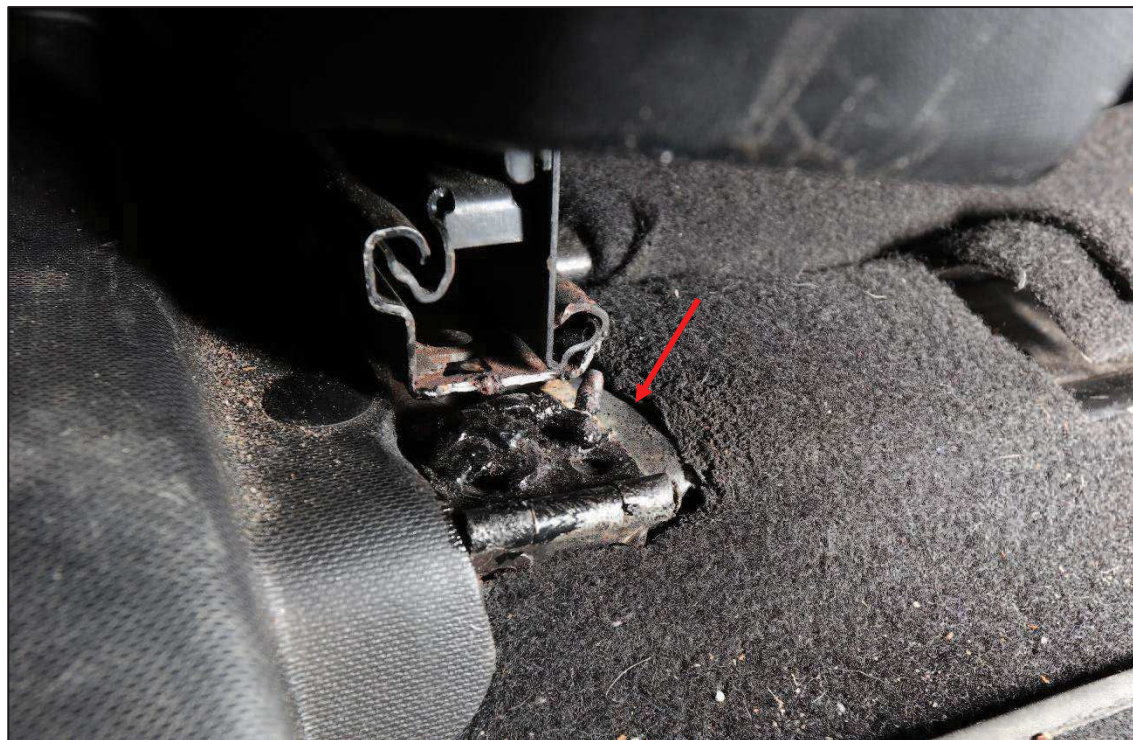
Figur 6. Foto av passagerarsätets främre högra sätesfäste, sett i fordonets färdriktning. Den röda pilen markerar det monterade gångjärnet.
