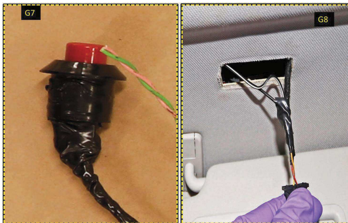
Figur 11: Bilden visar närbild på tryckströmbrytaren (G7) som satt vid rattstängan och kabelanslutningen (G8) på lampan ovanför solskyddet.
