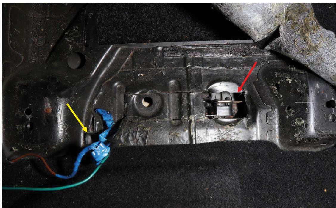
Figur 10. Foto från golvet under passagerarsätet. Den röda pilen markerar den fastmonterade låsanordningen och den gula pilen markerar kablarna (ses även i figur 8 ) som var anslutna till låsanordningen.
