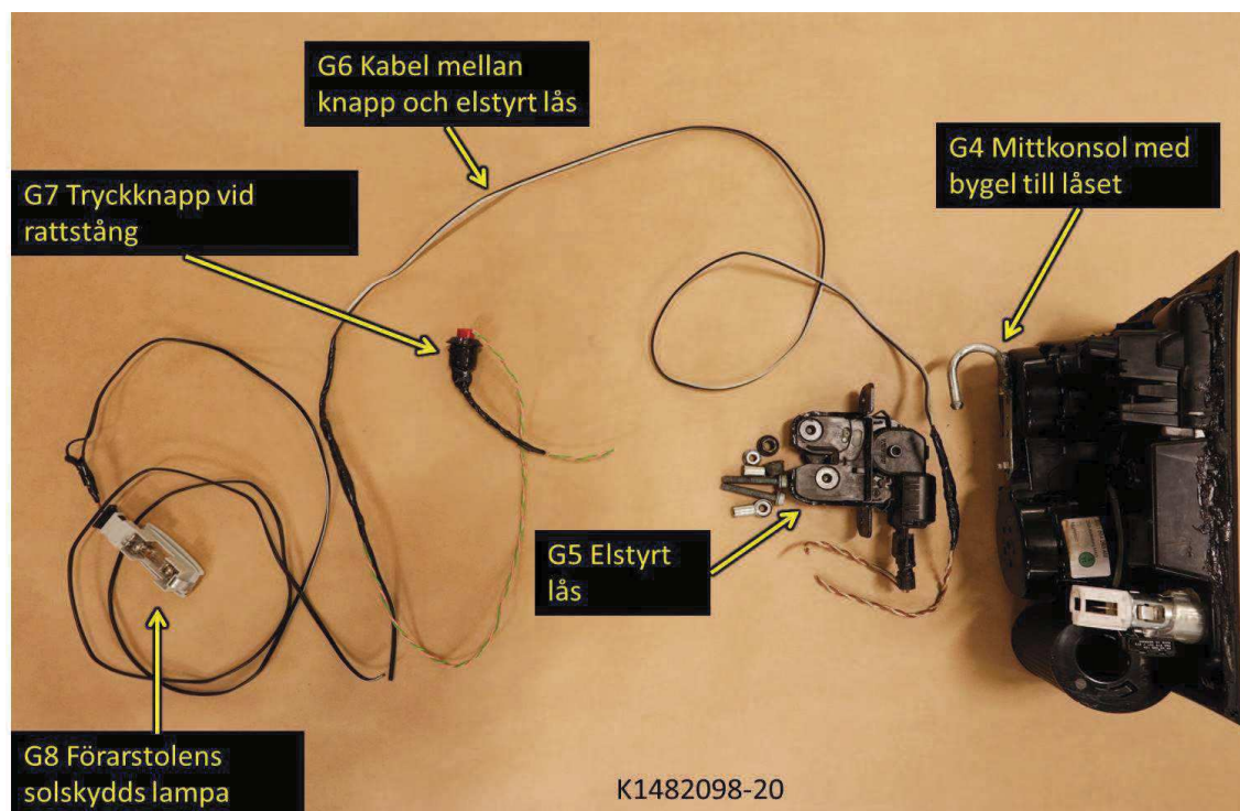
Figur 9: Bilden visar de kablarna, strömbrytaren och låsanordningen som monterades loss från bilen.
