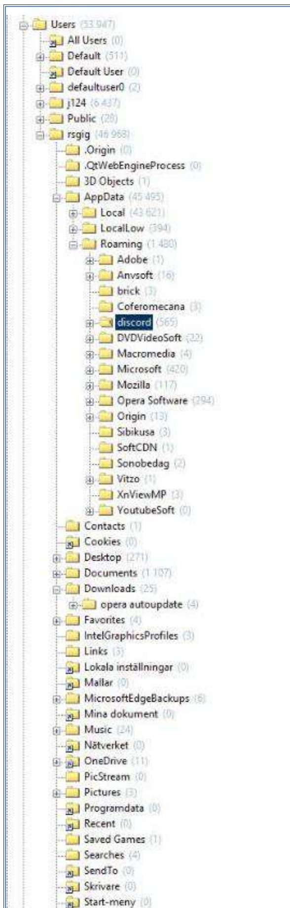
Bild 4. Katalogstruktur
