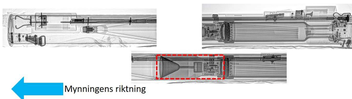
Bild 3: Beslagttaget pansarskott fotograferat i röntgen.
