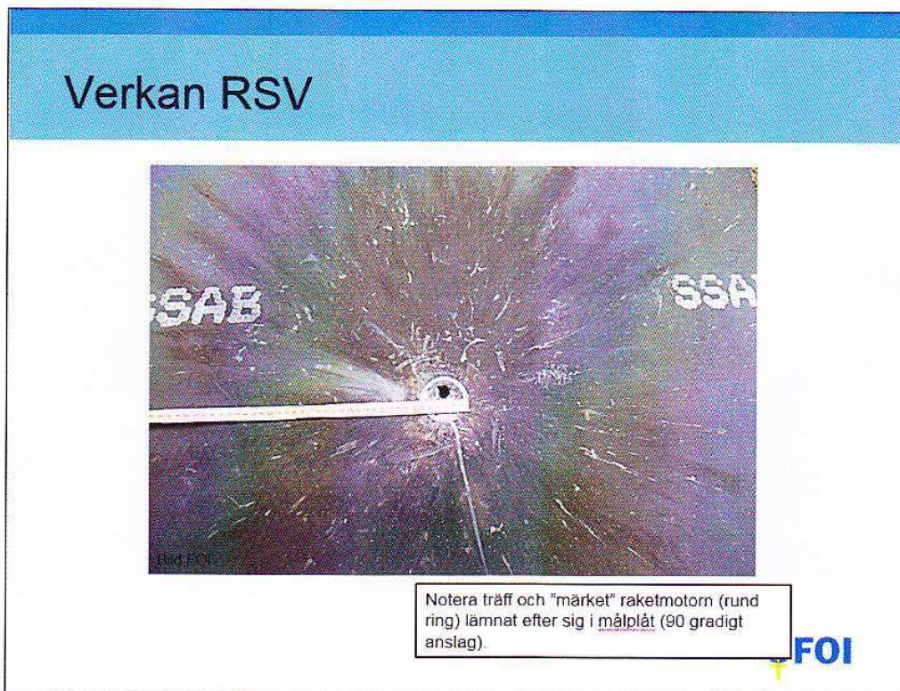
Figur 5: Verkan RSV. Genomgående hål i kraftig pansarplåt.
