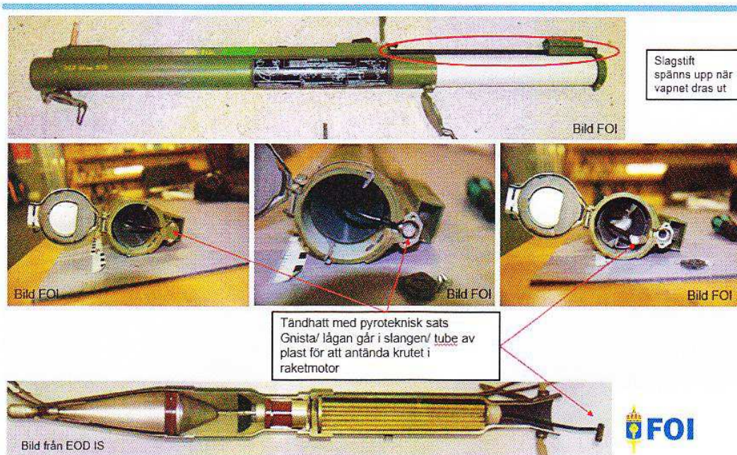
Figur 3: Detaljbilder av vapnet med utdraget bakre rör och raket. Tändhatten som påverkas av slagstiftet vid avfyring sitter i akterkant av röret. Pilarna pekar på tändhatten samt den svarta tuben/ plaströret som förmedlar sticklågan till raketkrutet i raketmotorn.
