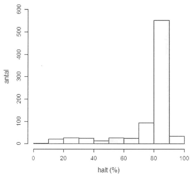
Figur 7. Histogram över kokainhalter i pulvermaterial som analyserats under 2023.
