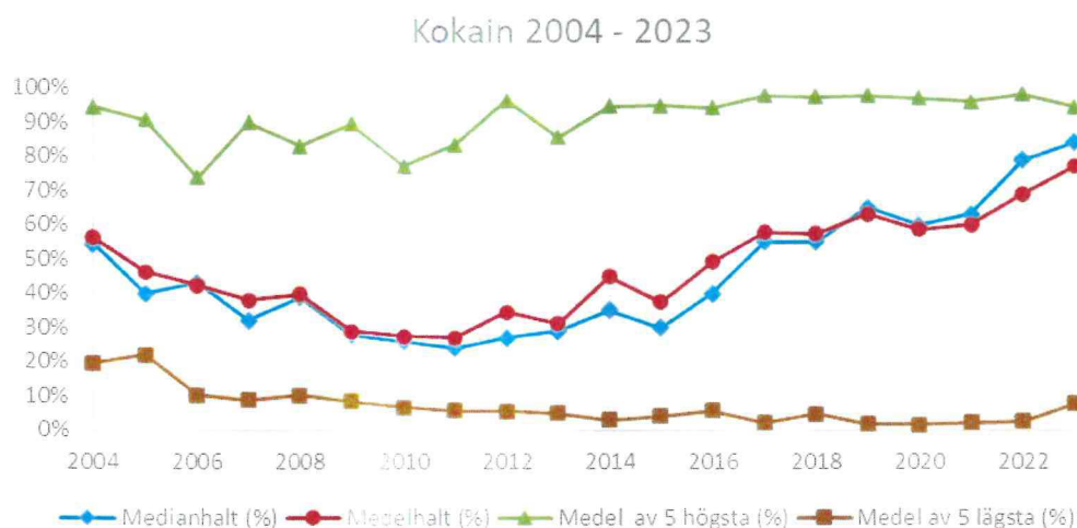
Figur 8. Diagram över kokainhalternas medelvärden, medianvärden samt medelvärden av de fem högsta och lägsta halterna i pulvermaterial för åren 2004–2023. Tabellerade värden för antal material, medel- och medianvärden samt medelvärden av max- och minhalter, se bilaga 6.2. Medelvärde har beräknats för halter om minst 1 %.
