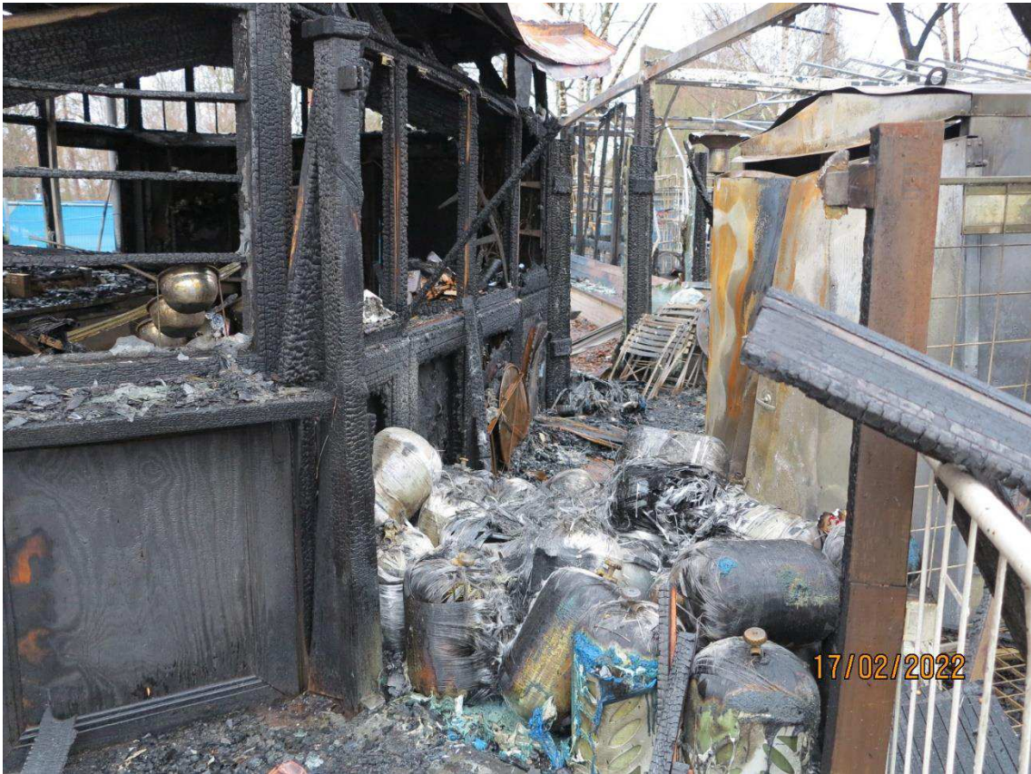
Figur 2. Bilden visar att stora mängder gasol förvarades intill baren oskyddade. Ett flertal av dessa flaskor rämnade (kompositflaskor) och bidrog avsevärt till den intensiva branden och en hög strålningsvärme. Foto: Åke Westman, 2022-02-17.
