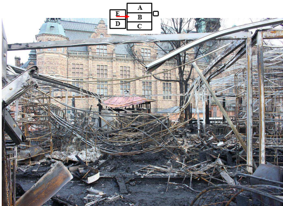
Figur 6. Sektion B sedd från den västra sidan. Här fanns företrädesvis de lägst belägna brandskadorna. I denna sektion var även ramverket som mest värmepåverkat/snedvridet och samtliga takstolar hade fallit ned mot marken. Röd pil på infälld orienteringsfigur visar ungefärlig fotoriktning.
