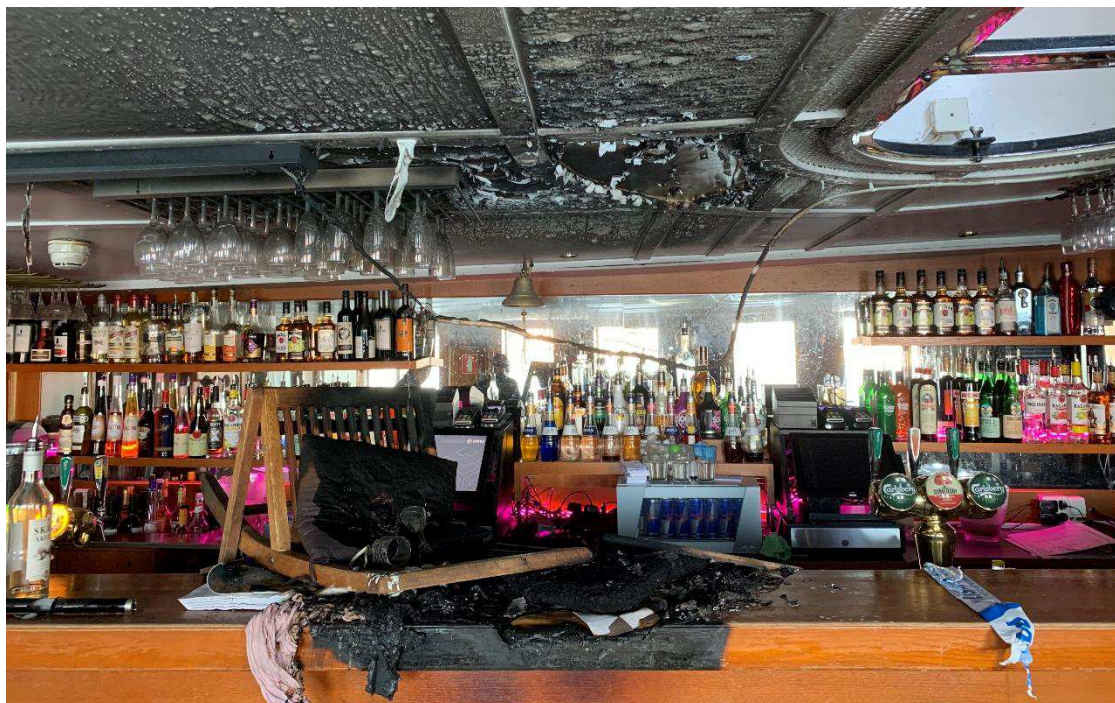
Figur 11. Delvis förkolnad kant till bardisken samt sotskador och värmepåverkan i taket ovanför bardisken.
