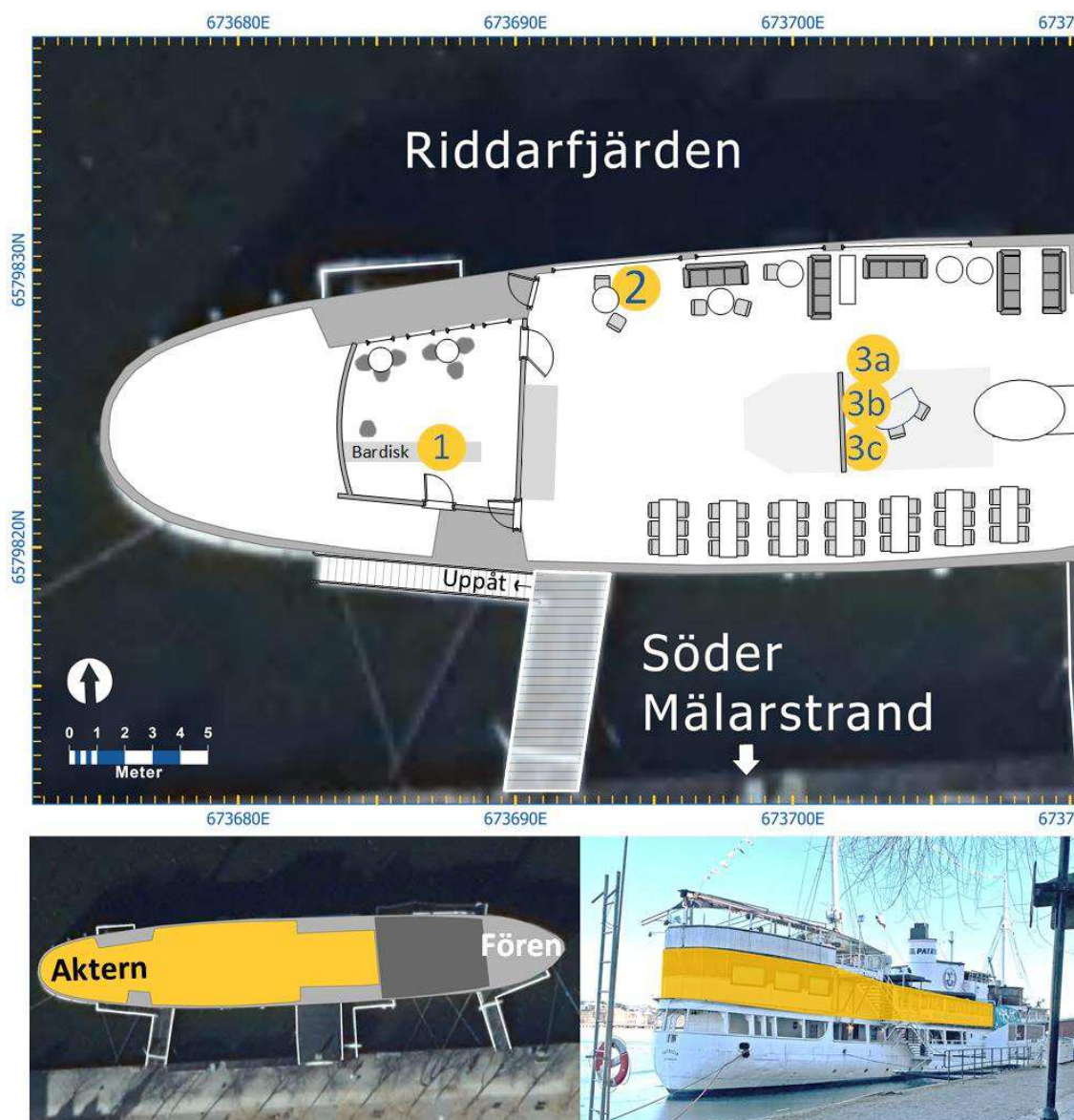
Figur 7. Bilden överst visar primära brandområden markerade med gula cirklar på planritning av Patricias restaurangdel. Gulmarkerade områden på de nedre bilderna visar planritningens utbredning. Strecken på kartramen: tjocka=5 meters avstånd; smala=0,5 meters avstånd. Baskarta Lantmäteriets ortofoton 2015-2021. Planritning koordinatsatt och bearbetad i ArcGis Pro med projektionen SWEREF99 TM.
