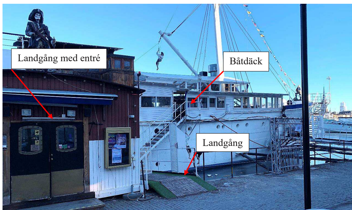
Figur 4. På mitten av båten var landgången med entré samt landgången bredvid där trappan gick upp till båtdäck. Fotograferat från kajen.
