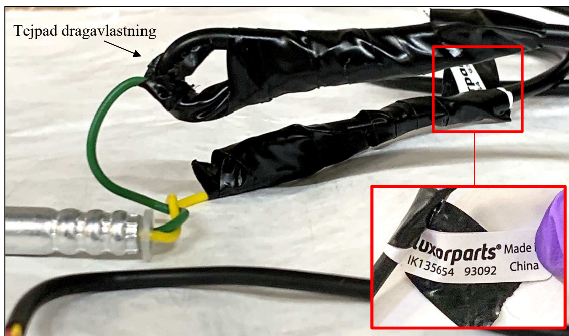
Figur 12. Tejpad dragavlastning på kopplingen mellan kabel tillhörande elsprängkapsel och svart förlängningskabel. Inflikad bild visar etiketten på ena kabeln.
