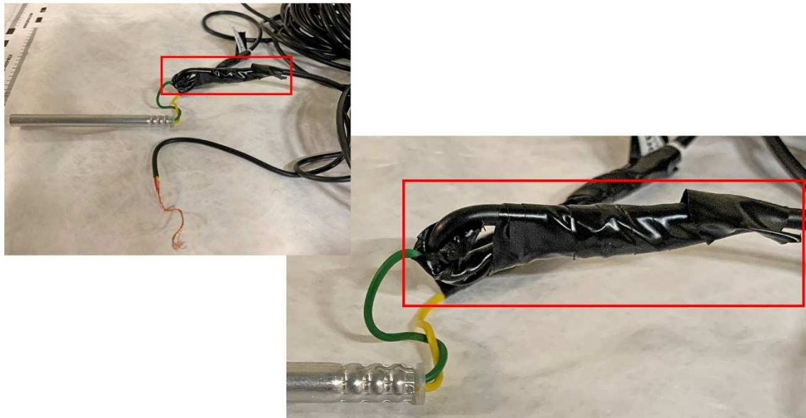
Bild 2: Detaljbild över den dragavlastade ihopskarvningen.
