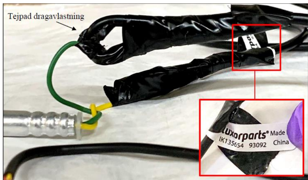
Figur 12. Tejpdragavlastning på kopplingen mellan kabel tillhörande elsprängkapsel och svart förlängningskabel. Inflikad bild visar etiketten på ena kabeln.
