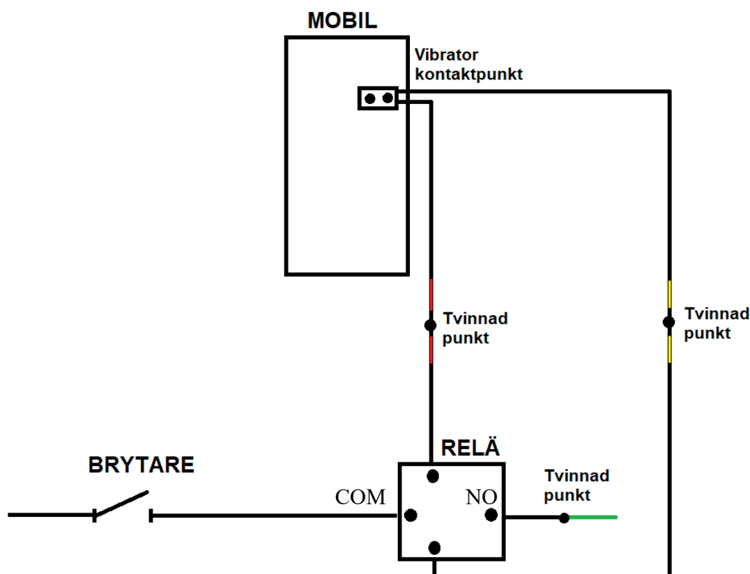
Figur 1. Skiss över kopplingen mellan BG92307-3 och BG92307-8.
