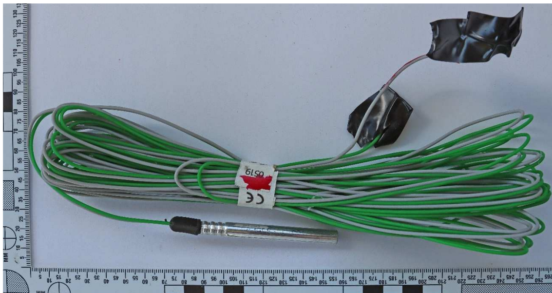
Bild 1: Beslagtagen elsprängkapsel.
