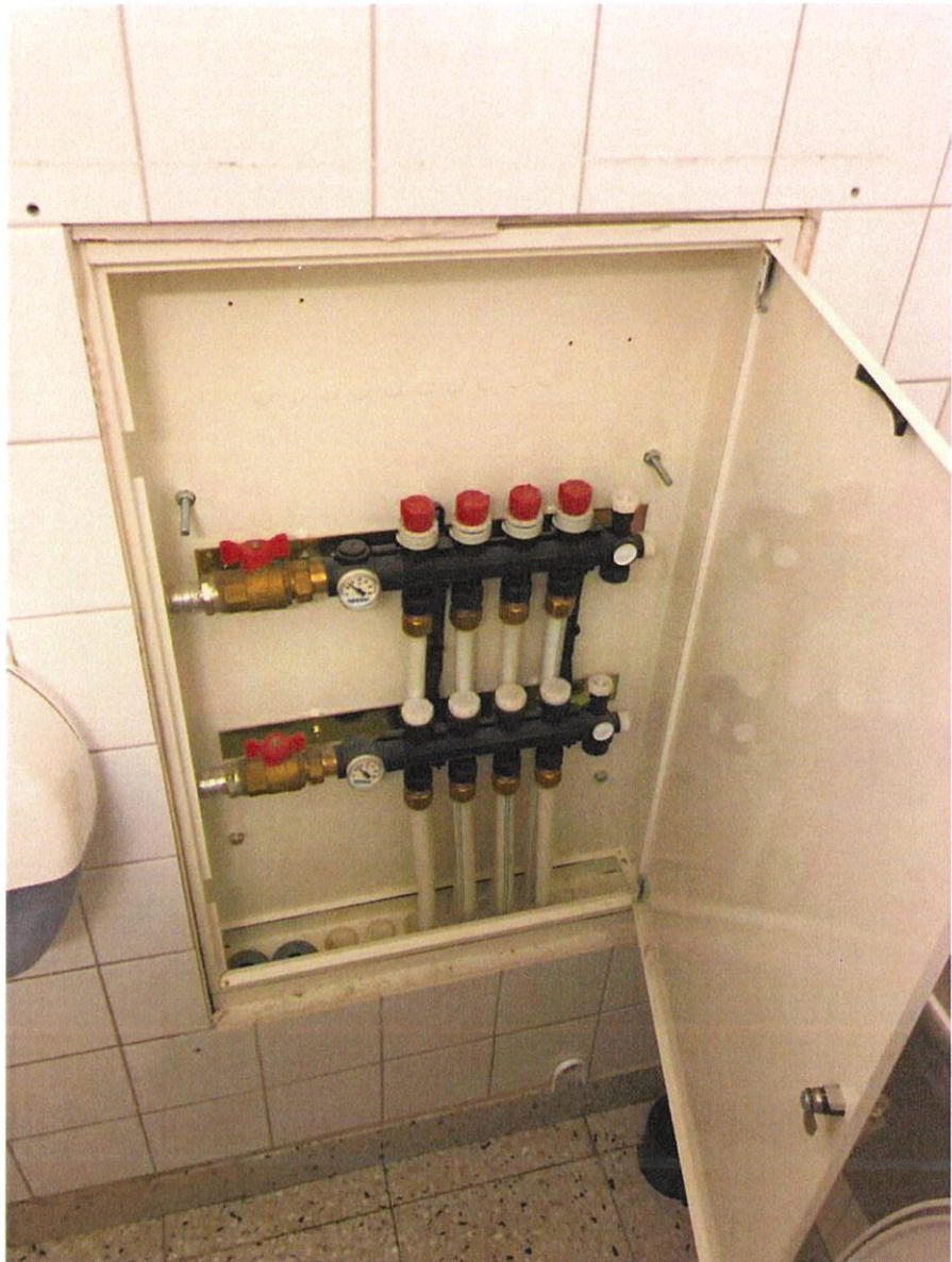
Vatteninstallation i plåtskåpet. Utrymmet är några centimeter djupt.
