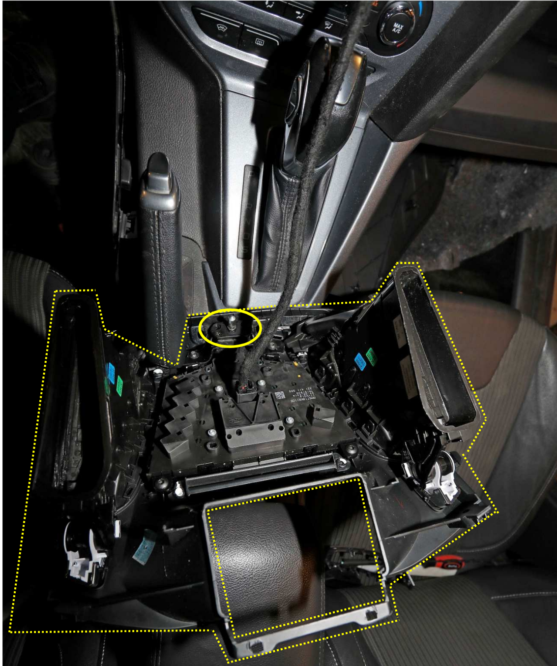
Figur 5. Instrumentpanelen är nedmonterad och ligger mellan framsätena, markerad med streckade linjer. Här är instrumentpanelens insida/baksida synlig. Cirkel markerar del av låsanordningen med låskolven som satt i låsanordningen i figur 4.
