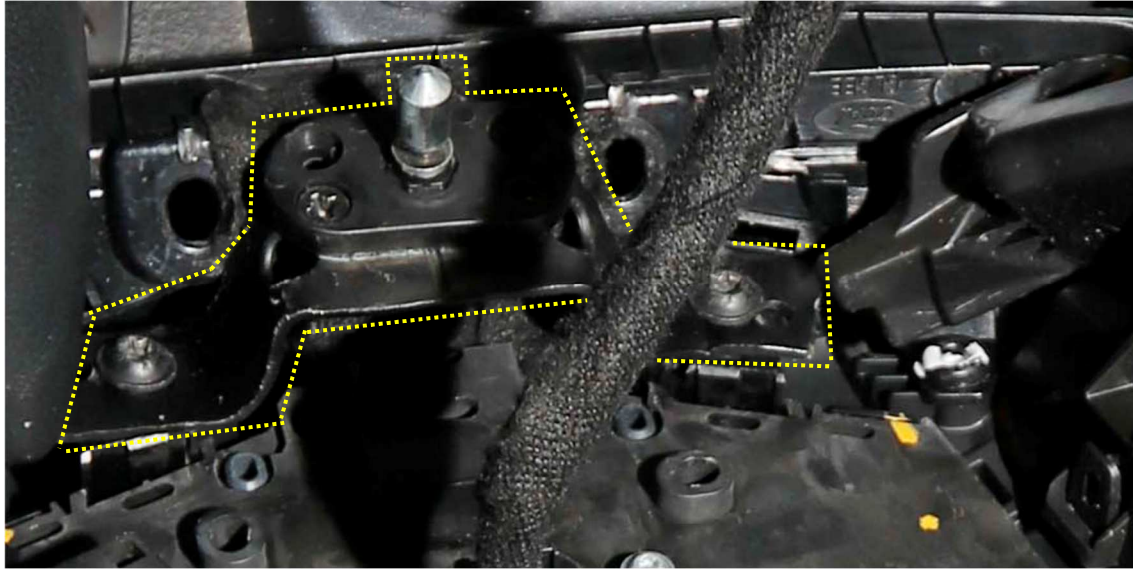
Figur 6. Närbild av del av låsanordningen med låskolvets fäste, på insidan/baksidan av instrumentpanelen, märkt med streckande linjer.
