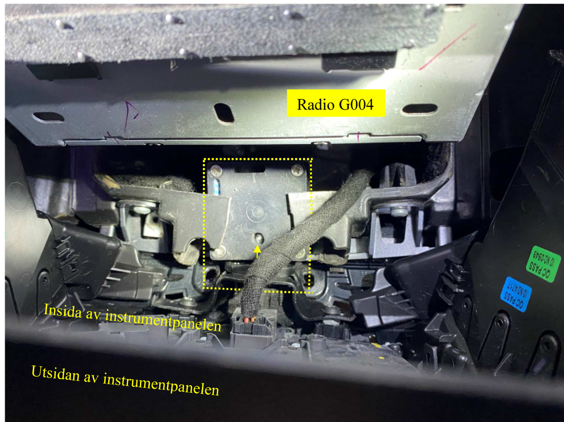
Figur 4. Fotograferat bakom/på insidan av den delvis bortmonterade instrumentpanelen, ned mot låsanordningen. Den nedre mörka delen av bilden är mot fordonets kupéutrymme och instrumentpanelens utsida. Den övre delen av bilden är på instrumentpanelens insida. Strecken markerar den låsta låsanordningen. Pilen markerar låskolven som iaktogs i hålet på låsanordningen.
