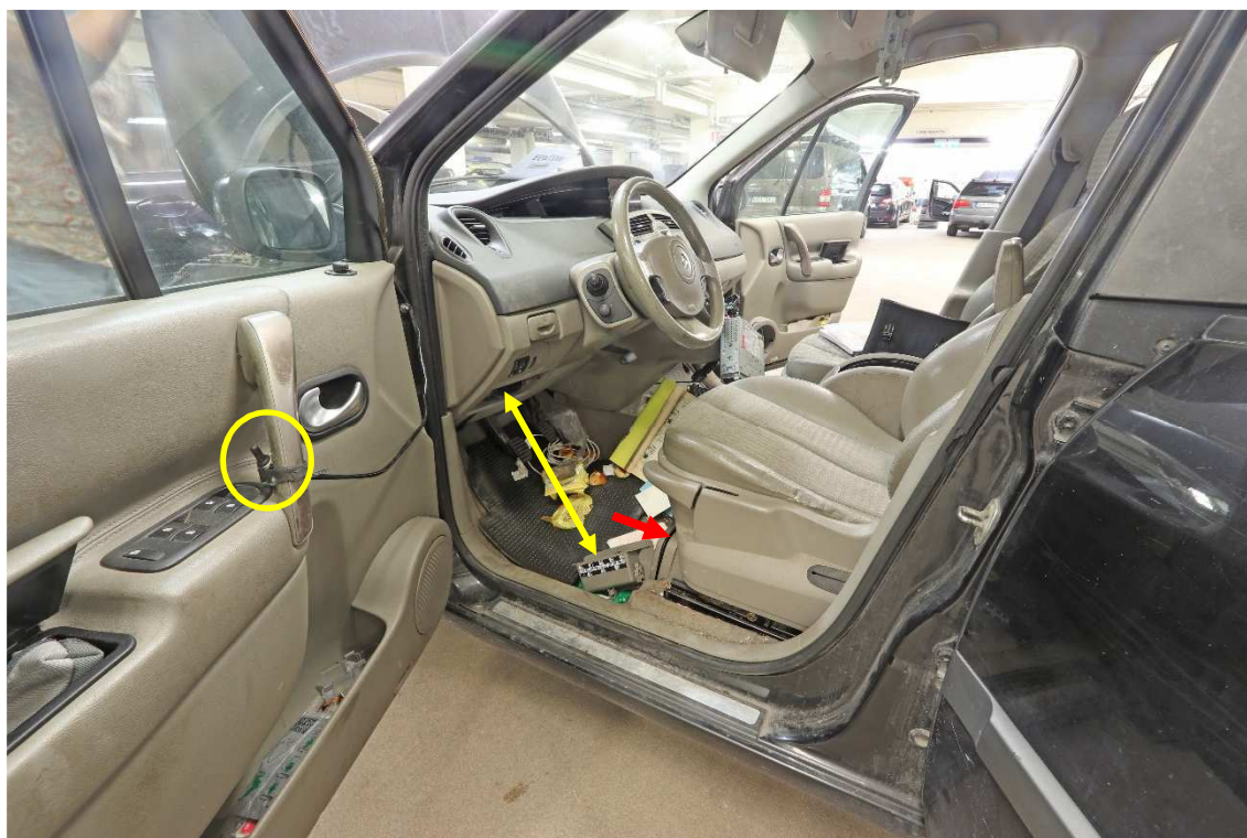
Figur 1. WZT493, Förarplatsen. Gul dubbelpil visar facket i panelen till vänster om ratten och lådan på golvet som tillhör facket. Röd pil visar placering för lådan under förarstolen. Switchknappen är markerad med gul cirkel.
