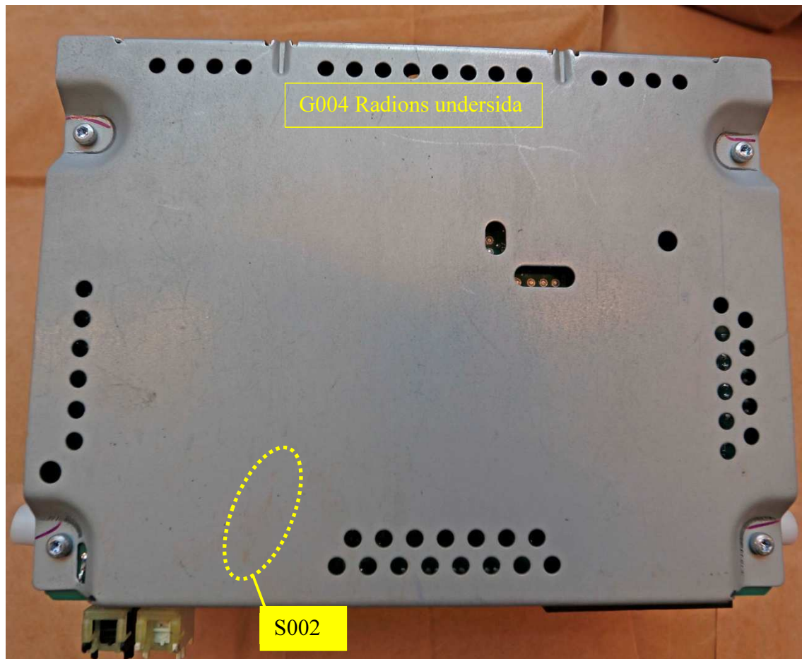
Figur 9. Cirkel markerar området där S002 säkrades på radions undersida.
