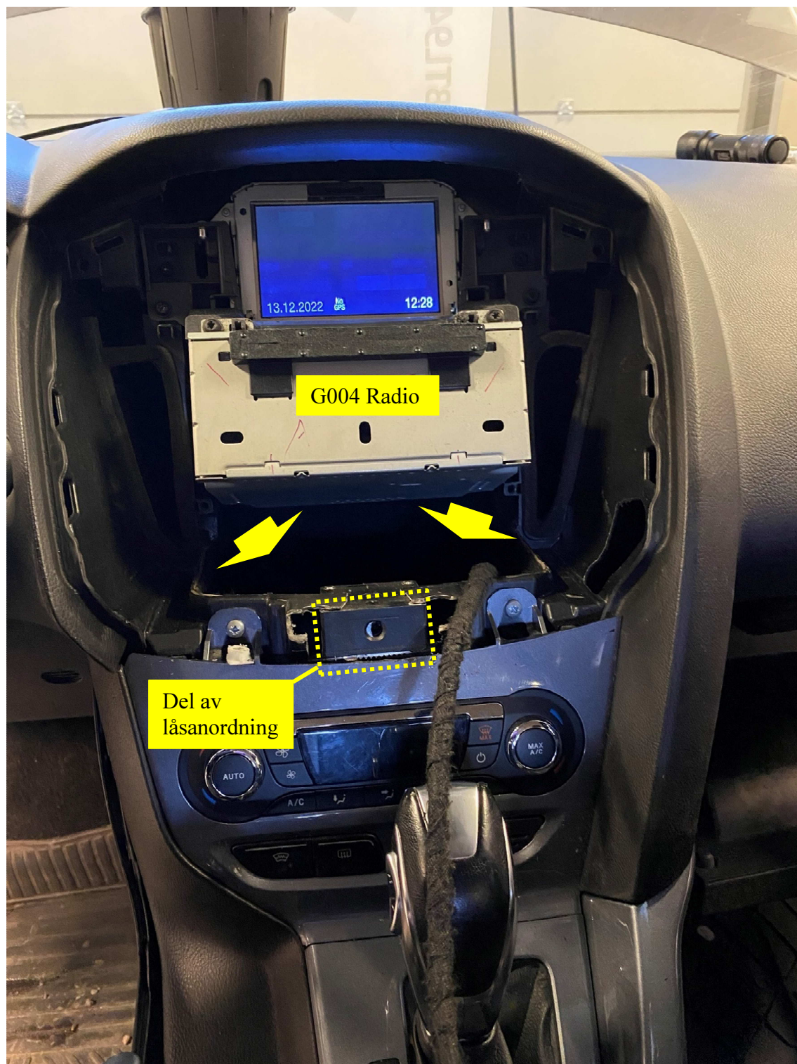
Figur 7. Mittkonsolen efter att instrumentpanelen monterats ned. Radion G004 är märkt. Pilarna markerar ingången till det filtbeklädda utrymmet. Rektangeln markerar del av låsanordning – där låskolven ska fästa för att låsa.
