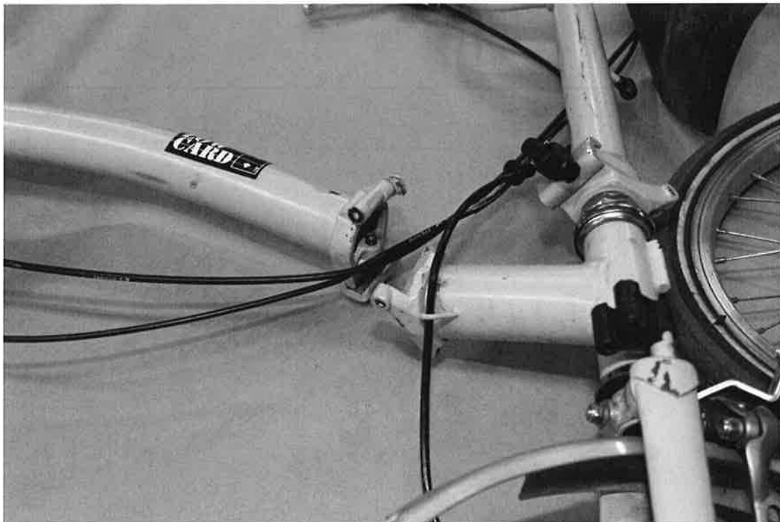
Bild 18. Detaljbild på brottytan vid det övre ramröret.
