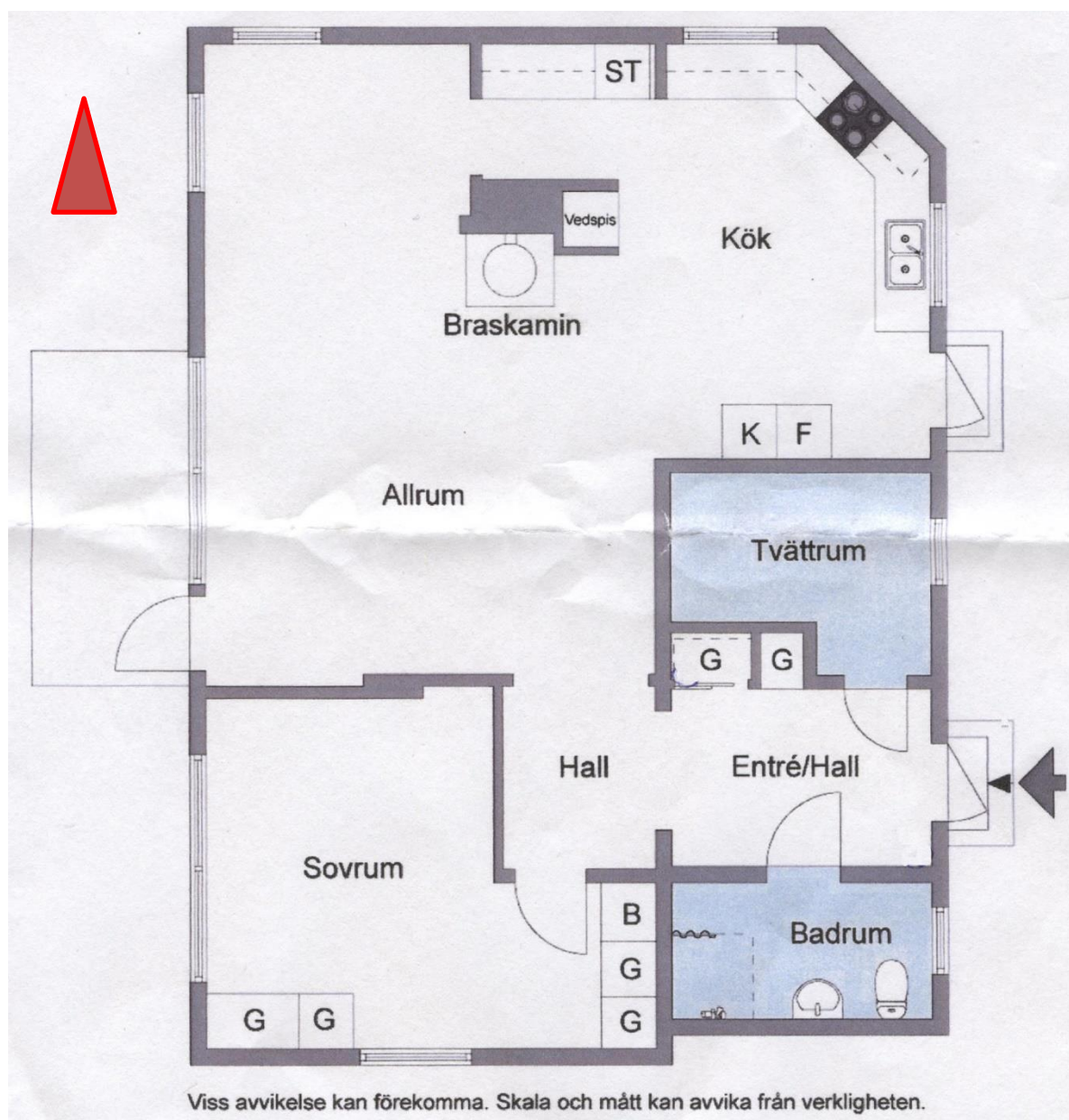
Bild 8 en planskiss över huset vilken vi fick av fastighetsägaren (för övrigt granne med aktuellt hus). Den röda pilen pekar åt norr.
