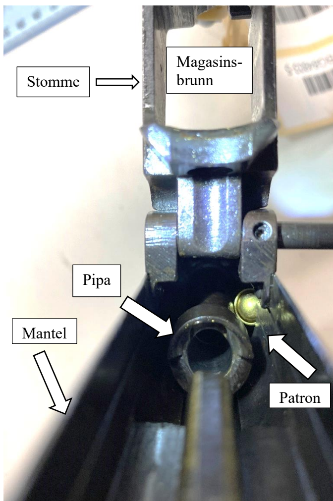
Figur 6. Patron mellan pipan och manteln på materialet BG84803-5
