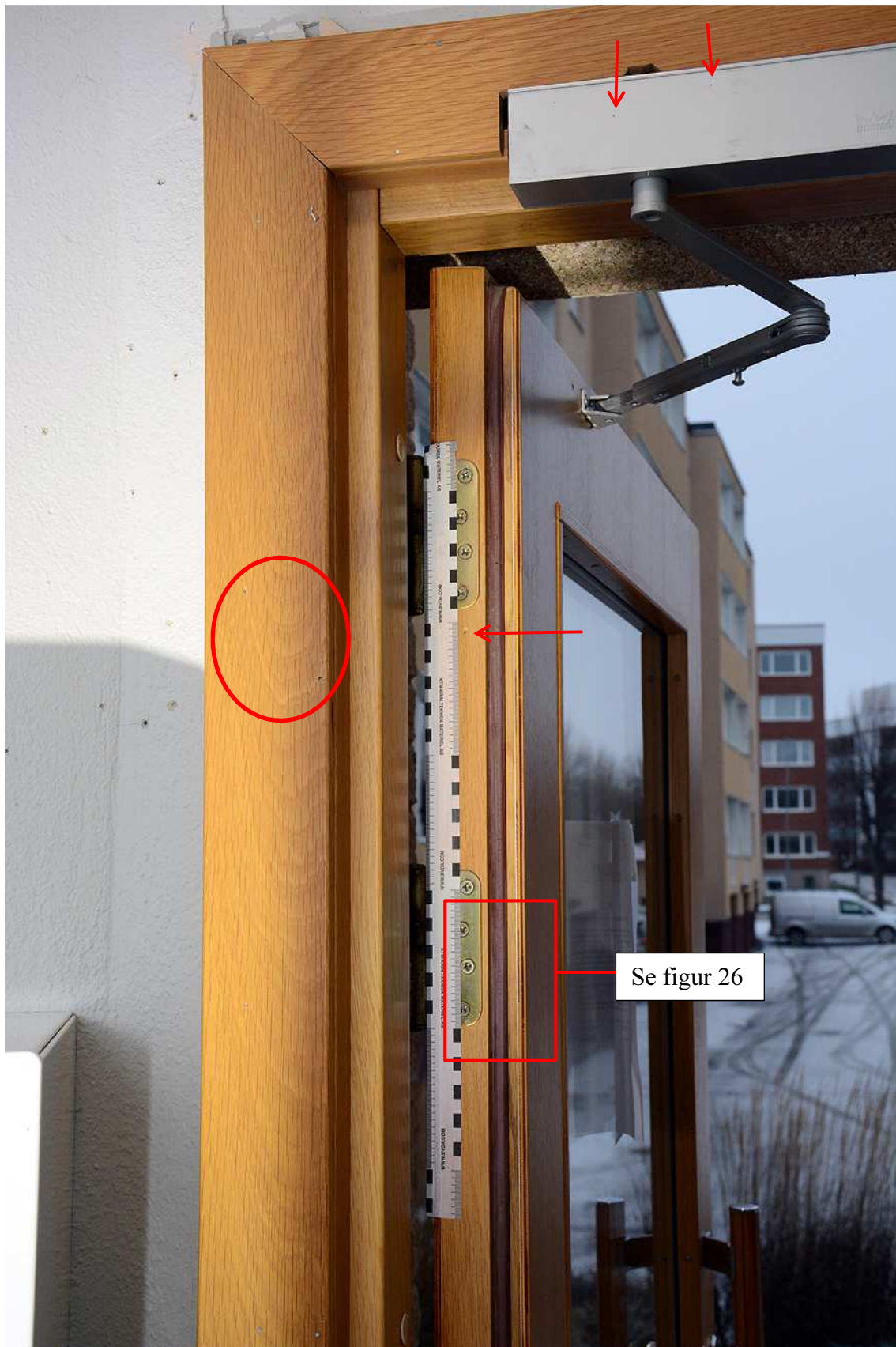
Figur 25. Entrédörren i uppställt läge. Skador sannolikt orsakade av stålkulor markerade. På väggen till vänster om dörrfodret ses ett tiotal liknande skador.
