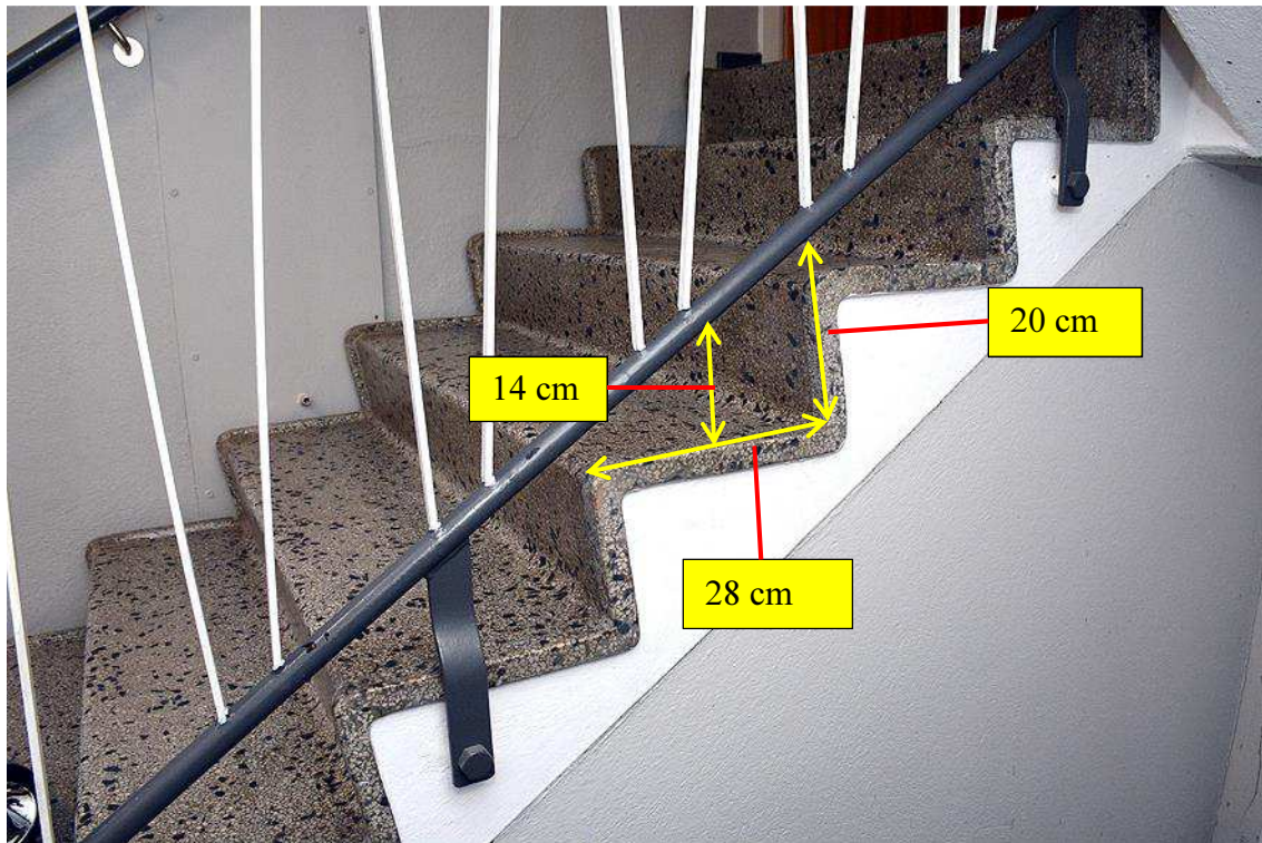
Figur 27. Mått trappsteg och trappräcke.
