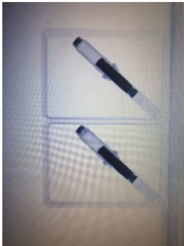
3. 2020-12-14 Blå vägen 32, Björklinge. Röntgen av sprängkapsel efter desaptering.
