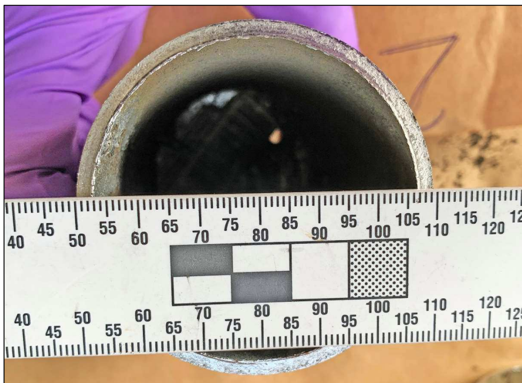
Figur 14. Tjockleken var densamma på båda rören (3 mm). Detta är rörbomb 2. Längst ned i botten av röret skymtas etiketten som ses närmare i figur 15.
