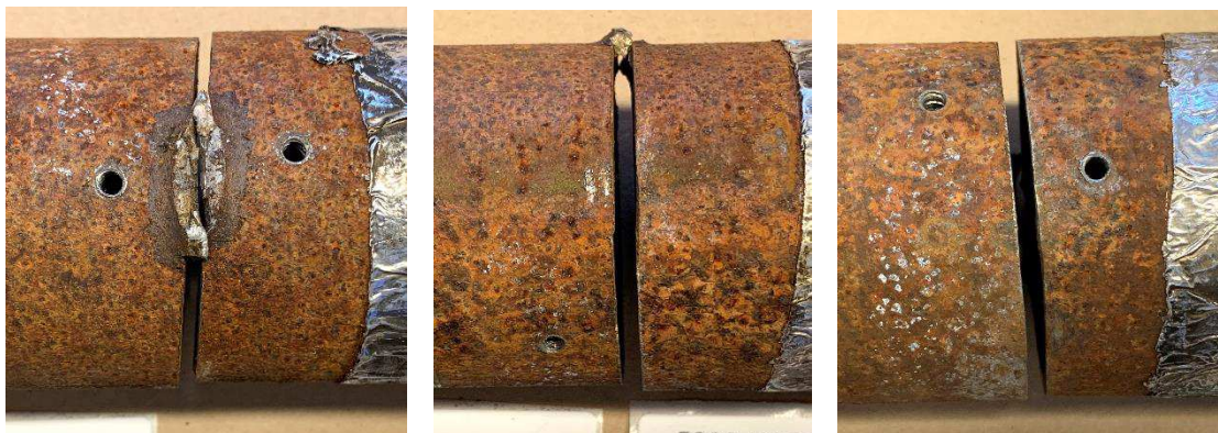
Figur 2. Rördel BG99160-1:1/2 till vänster och rördel BG120241-1:2 till höger i respektive bild. Förstoring på snittet mellan rördelarna sett från tre olika vinklar.
