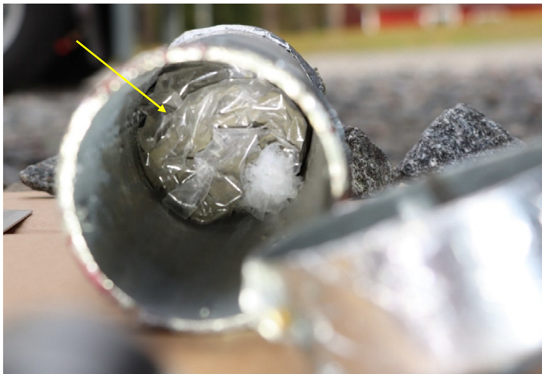
Figur 5. Metallröret i genomskäring. I botten syns plastpåsen med pyroteknisk sats vilken är markerad.
