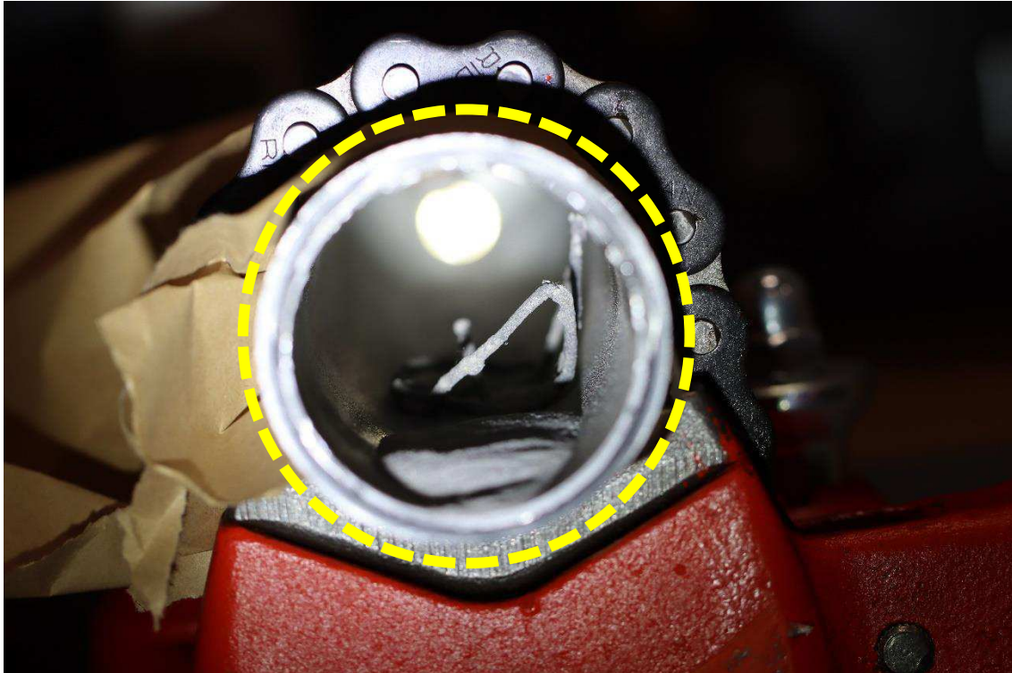
Figur 5. Gasflaskan (BG94665-1) markerad i bild och fotograferad efter det att den skurits upp av bombtekniker och större delen av pulvret i flaskan tömts ut. Inuti ses en del kvarvarande pulver samt den egentillverkade krutstubintråden (S011).
