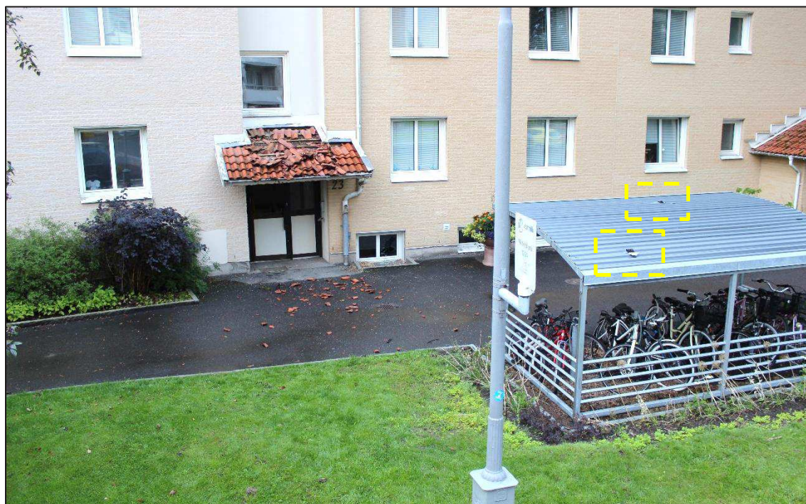
Figur 4. Krossade takpannor låg utanför entrén och taket ovanför hade skador. Skador i taket till cykelskjulet markeras med rektanglar.
